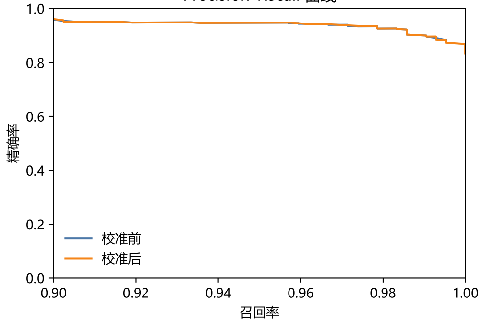
Precision-Recall 曲线
