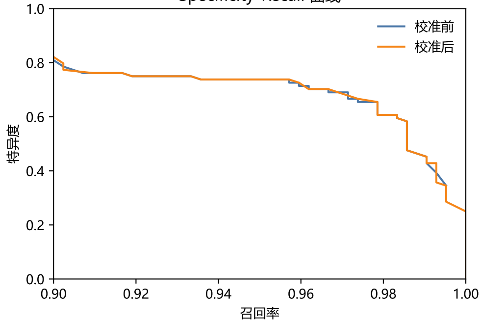
Specificity-Recall 曲线
