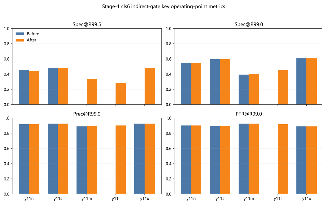
图 3 六类间接 gate 五模型的关键锚点指标对比
