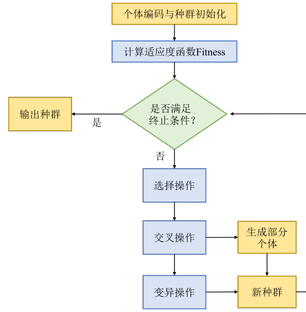
图 13 遗传算法流程图
