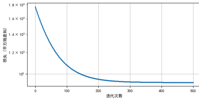
图 7: 高斯-牛顿迭代误差收敛情况
