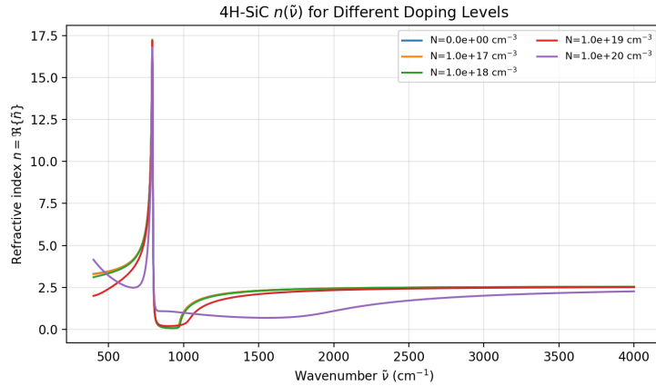
图 1: 碳化硅材料在给定掺杂浓度下折射率 (实部) 随入射光波数的变化曲线
