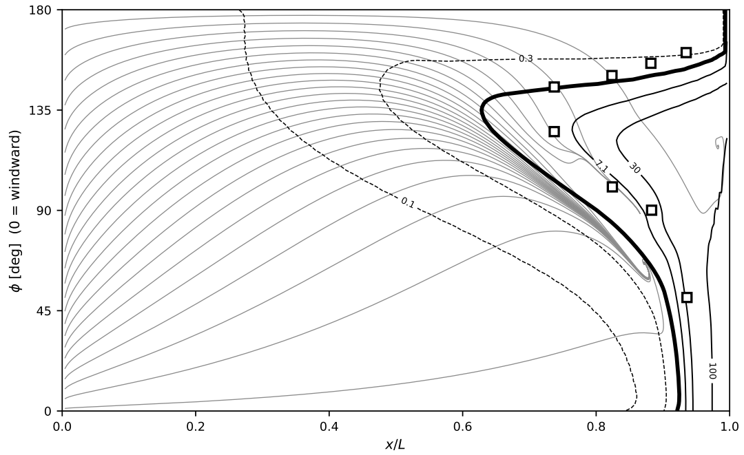
Fig. 26 \alpha = 5^\circ , Re_L = 1.52 \times 10^6 .
