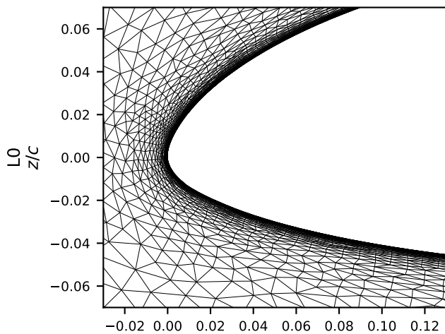
Leading edge
