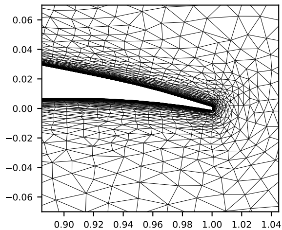
Trailing edge
