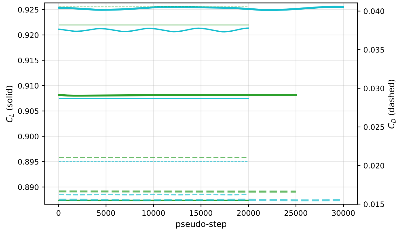
\alpha=7^\circ : C_L , C_D
