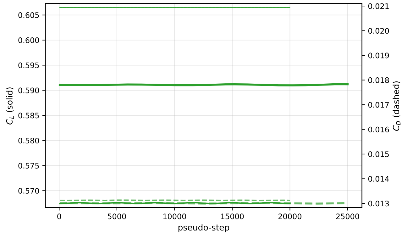
\alpha=2^\circ : C_L , C_D
