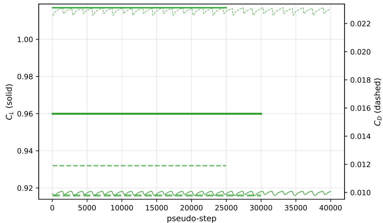
\alpha=4^\circ : C_L , C_D
