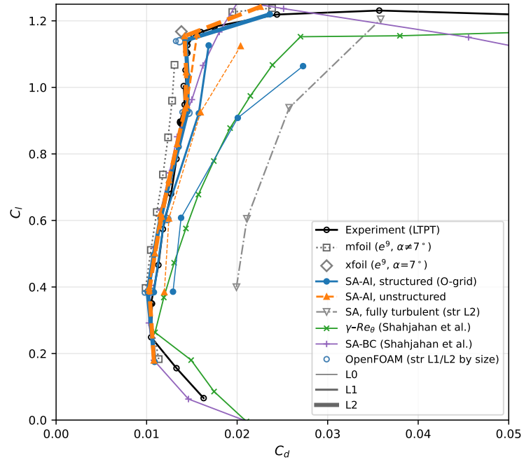
Figure A13: Eppler 387 drag polar.
