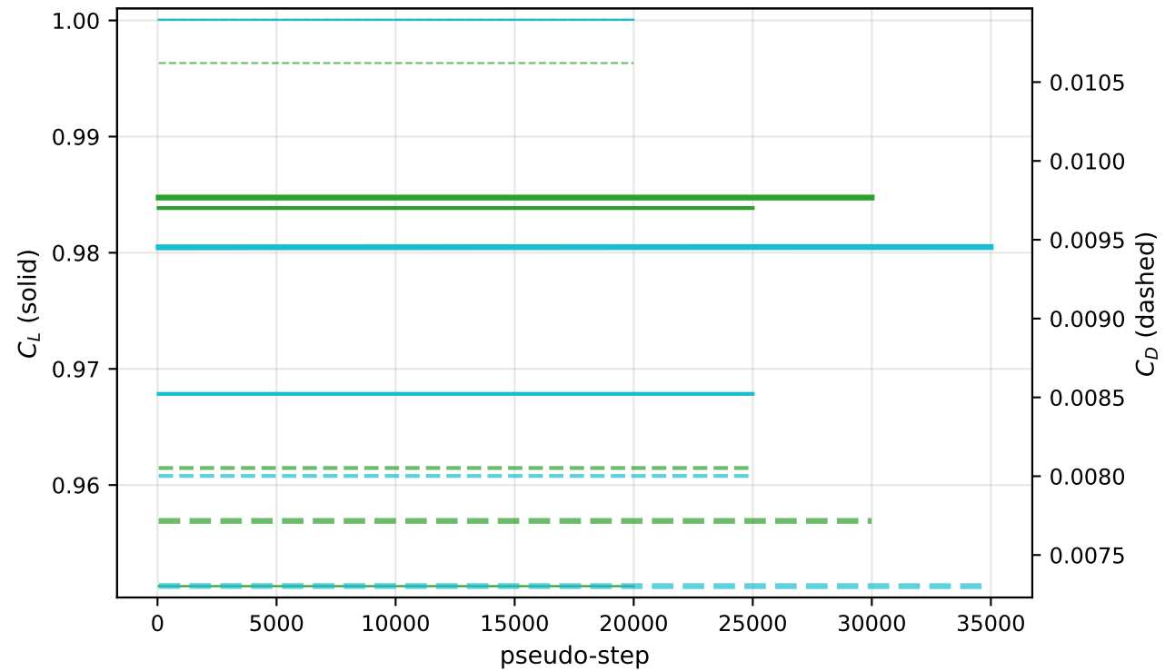
\alpha=4^\circ : C_L , C_D
