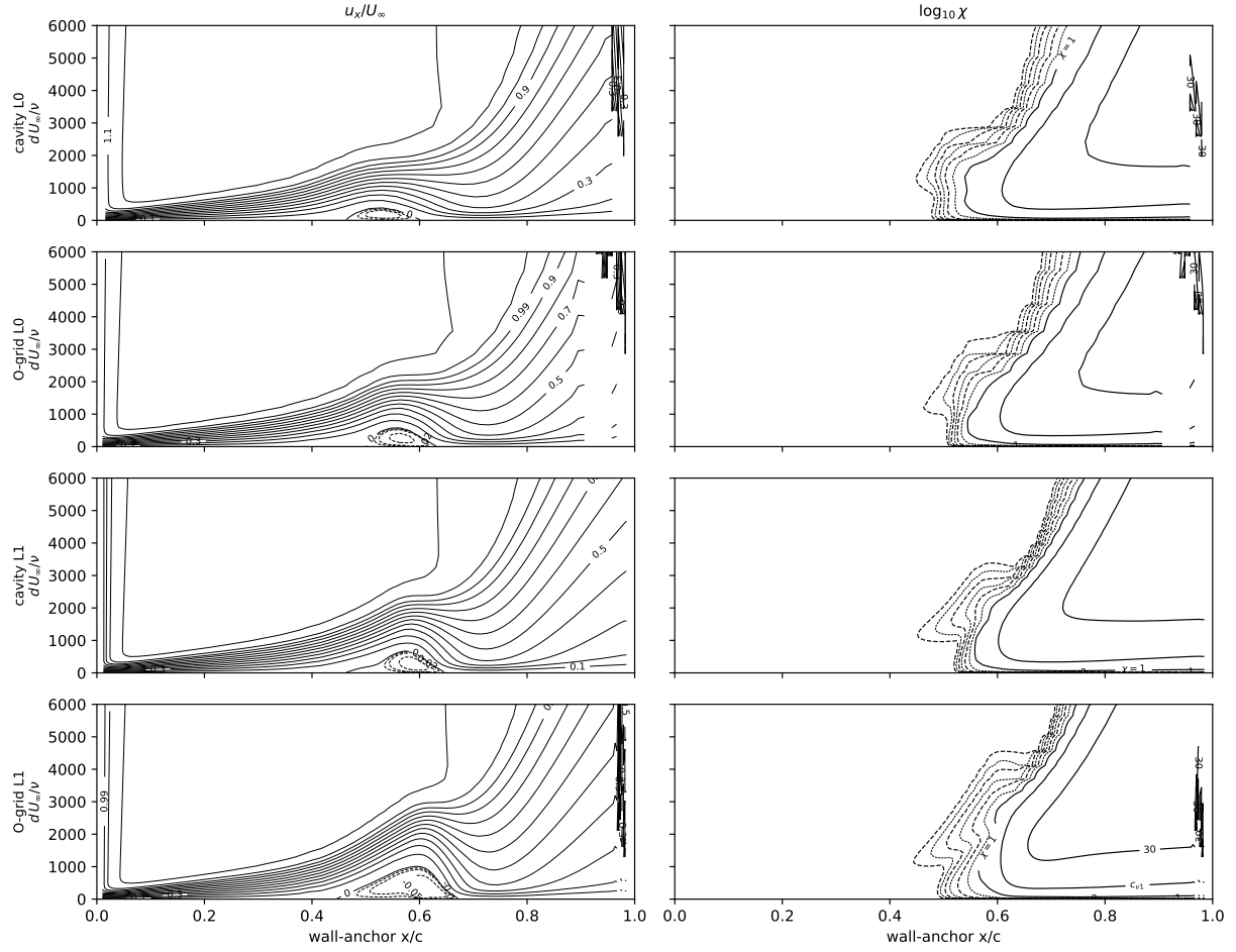
Fig. D14 As Fig. D12, at \eta = 0.92 .
