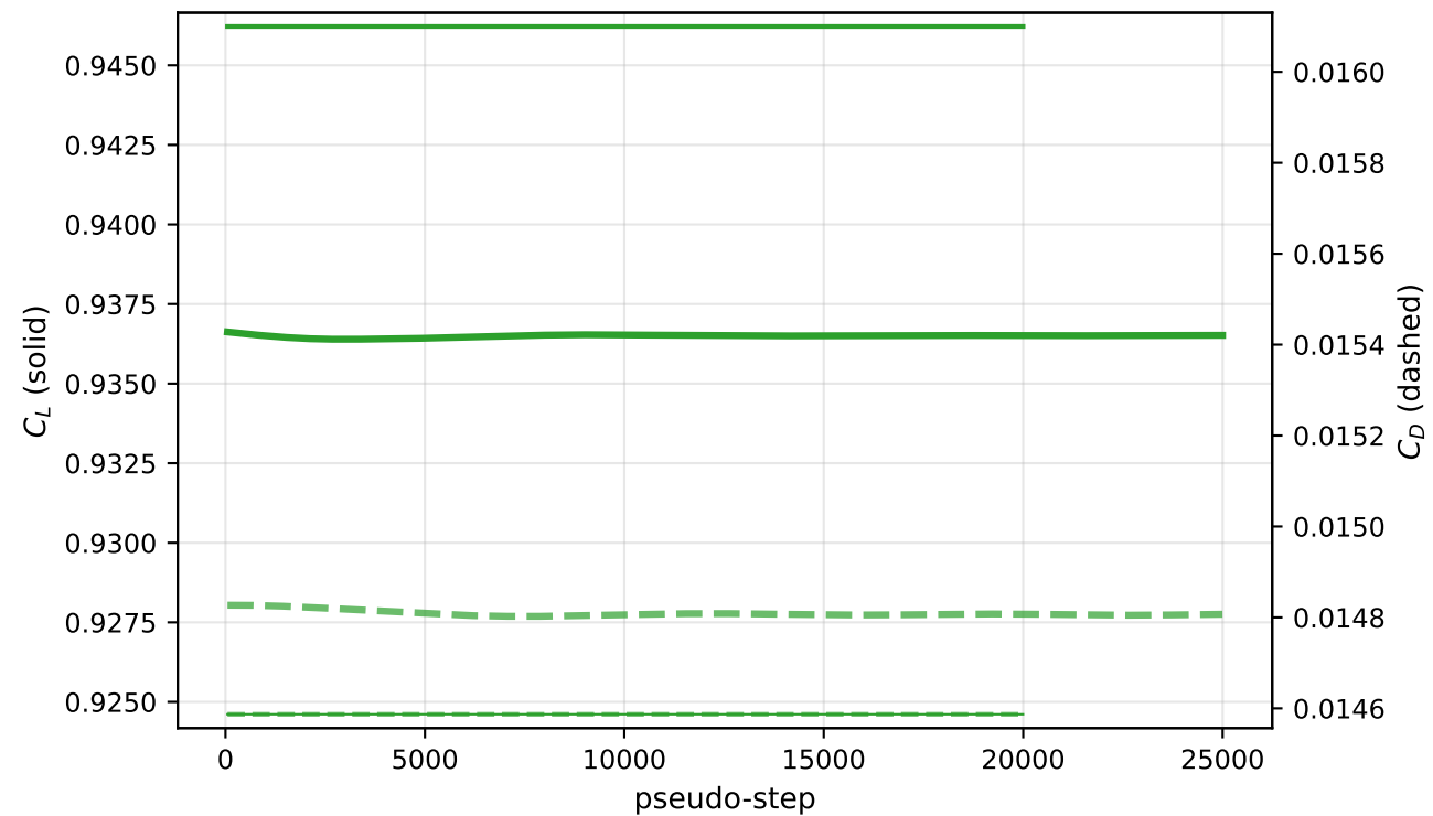
\alpha=7^\circ : C_L , C_D
