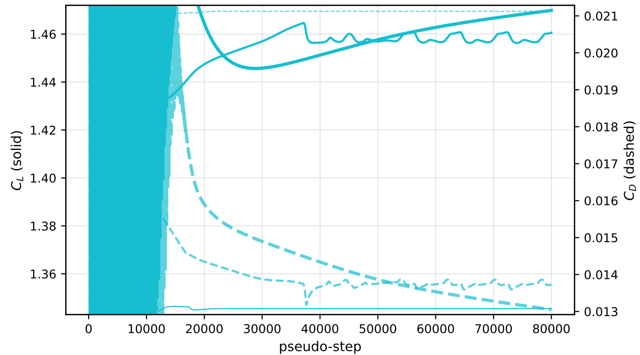
\alpha=15^\circ : C_L , C_D
