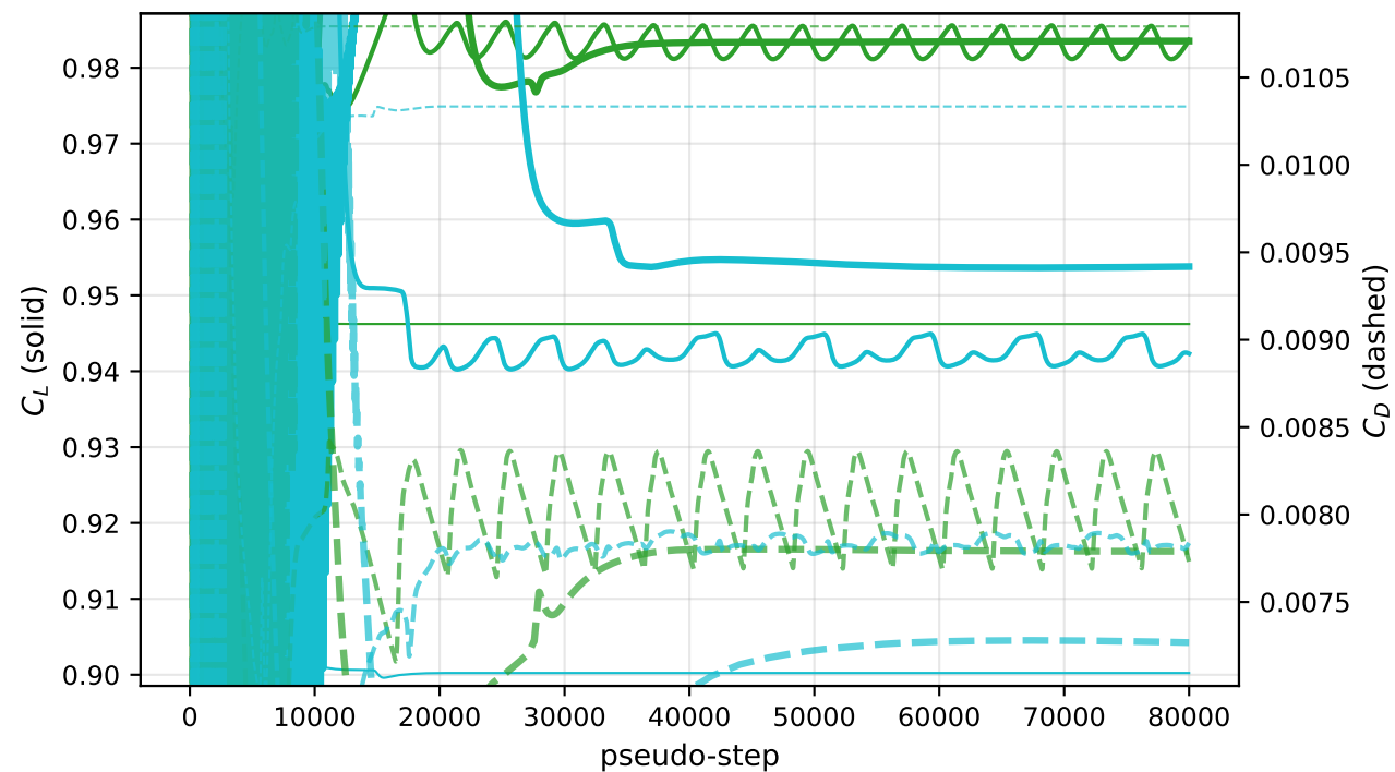
\alpha=4^\circ : C_L , C_D
