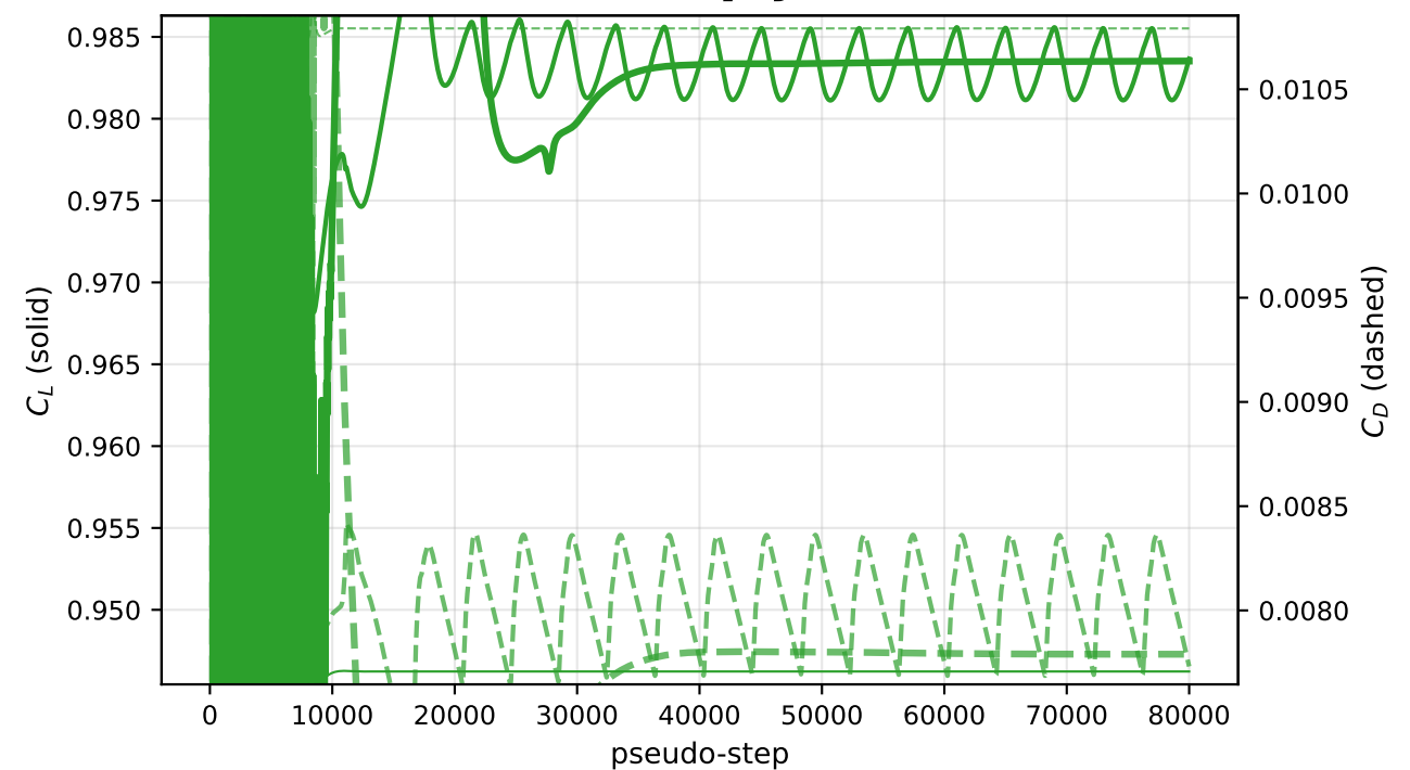
\alpha=4^\circ : C_L , C_D
