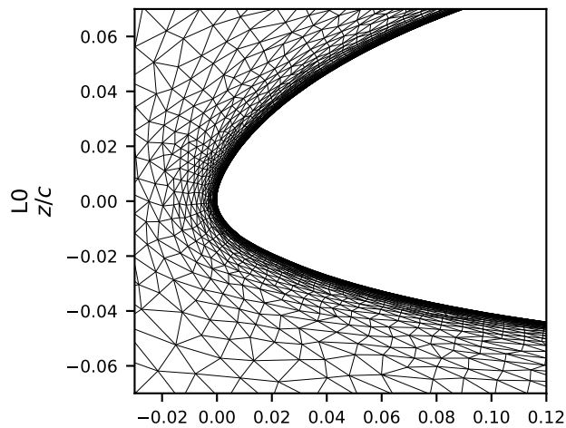
Leading edge
