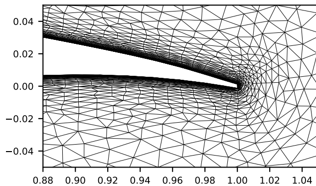
Trailing edge
