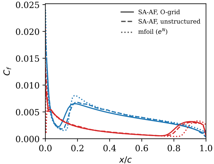
C_f, \alpha = 4^\circ
