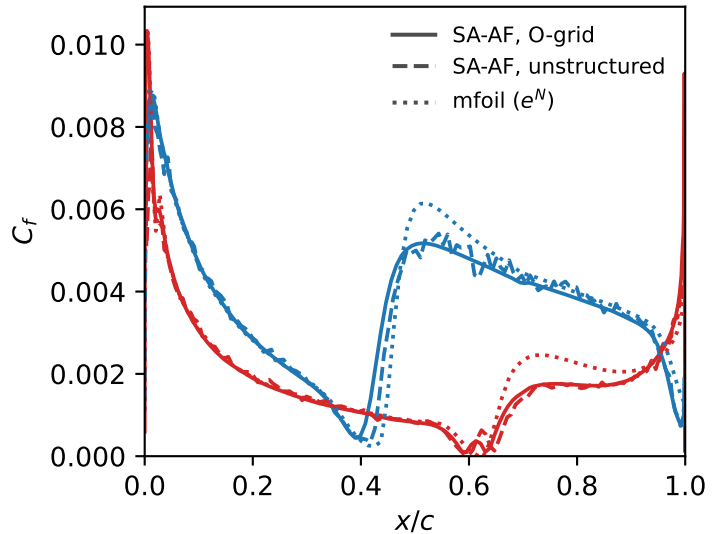
C_f, \alpha = 0^\circ
