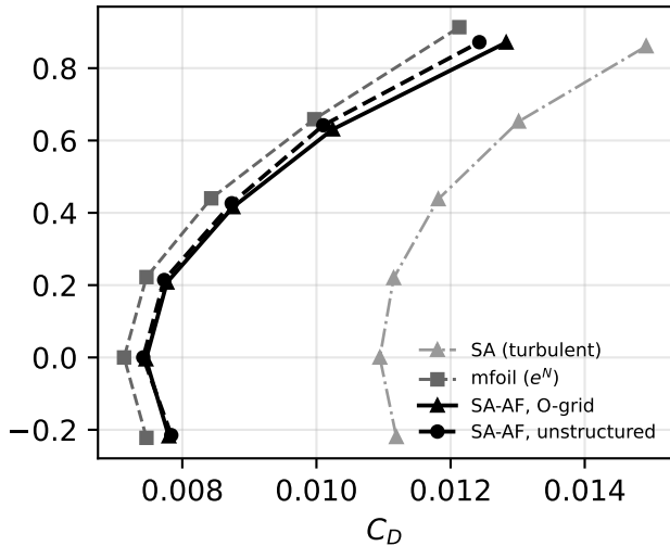
NACA 0012
