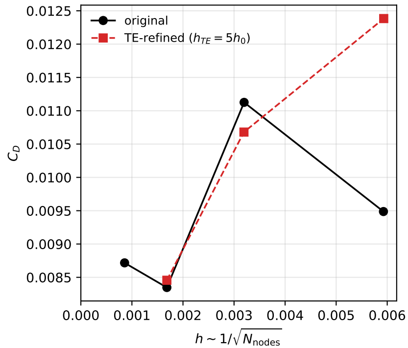
(b) drag
