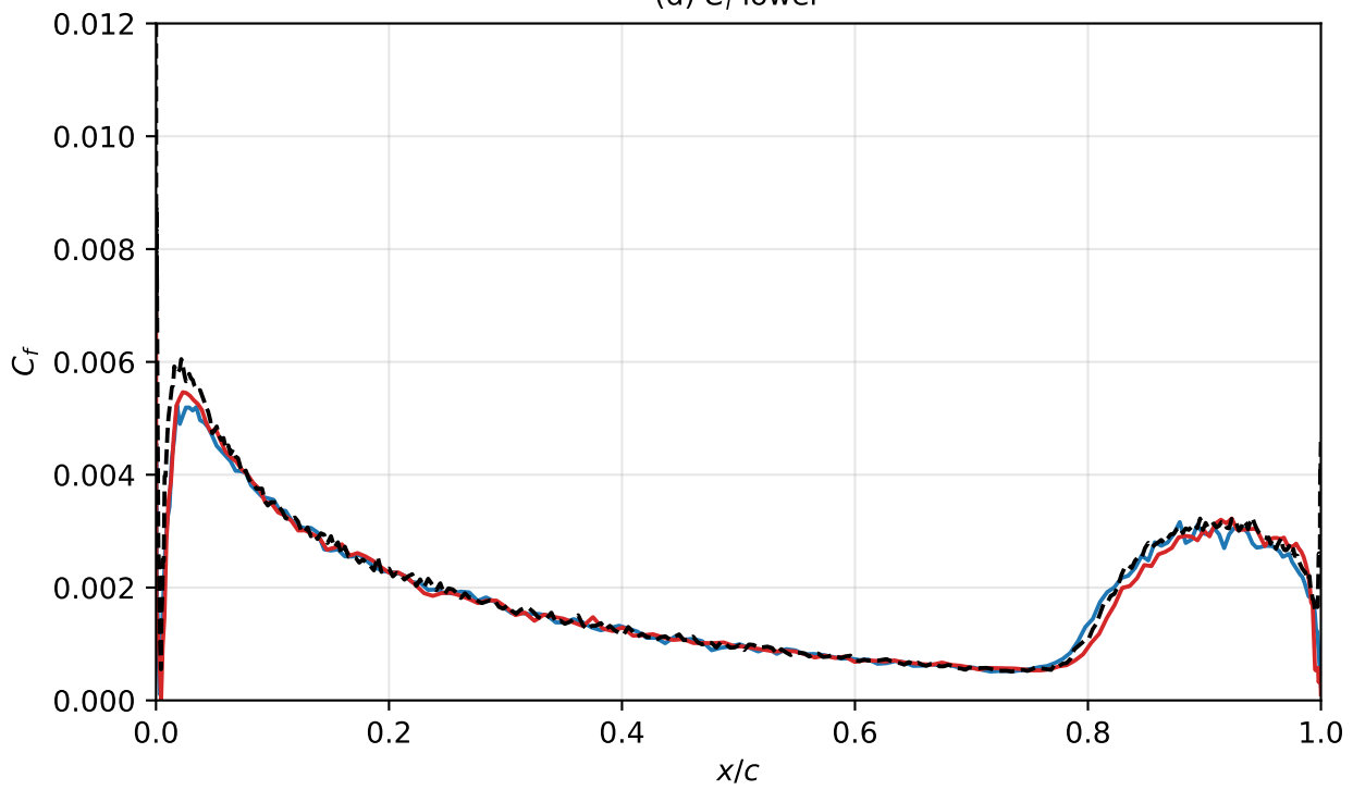
(d) C_f lower
