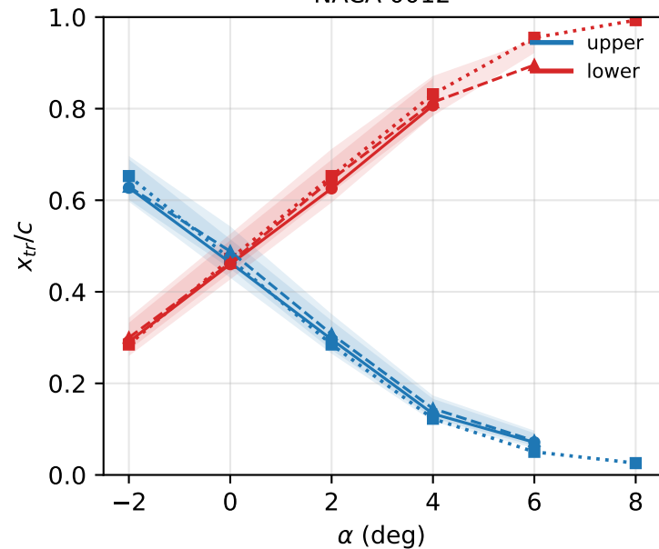
NACA 0012
