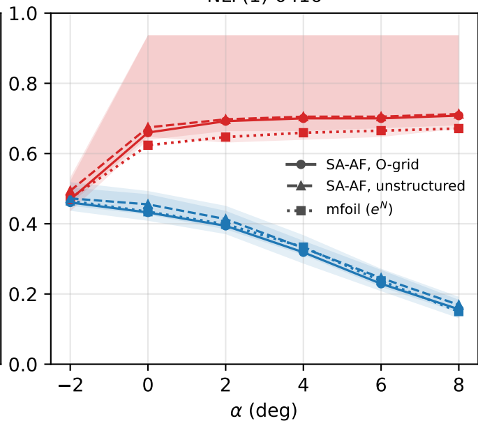
NLF(1)-0416
