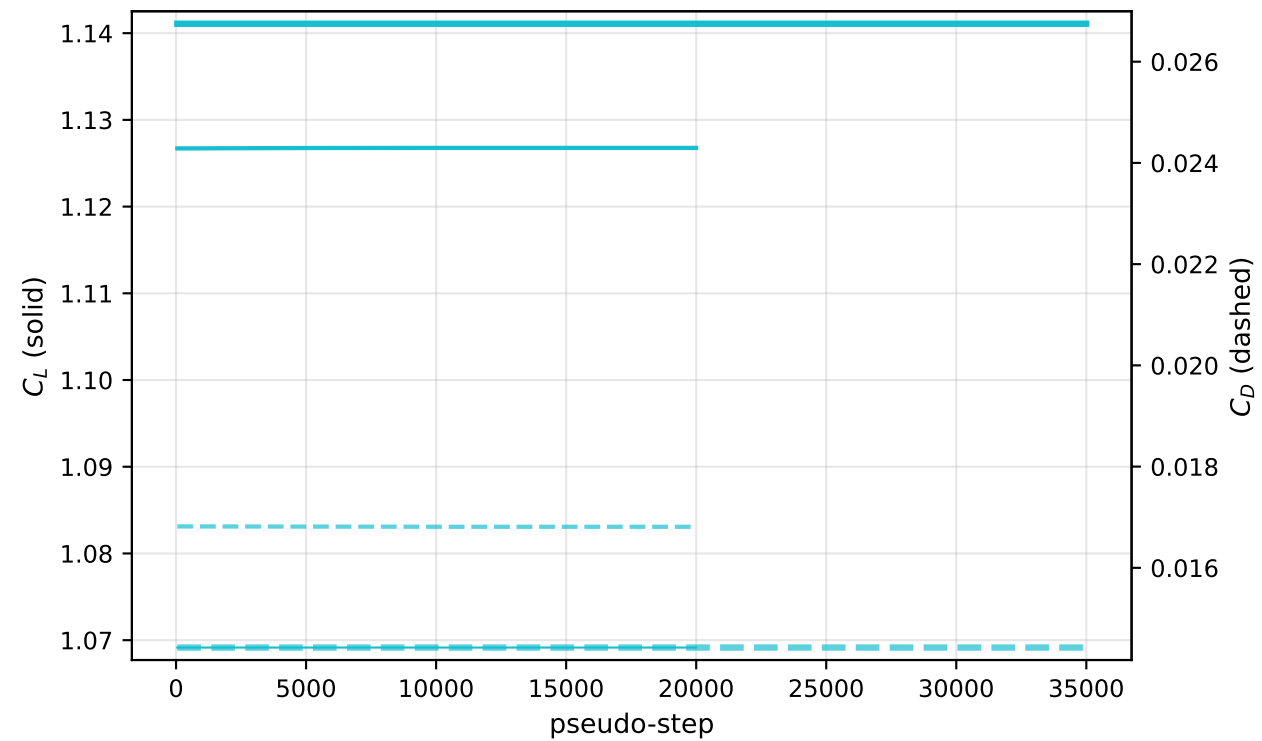
\alpha=7^\circ : C_L , C_D
