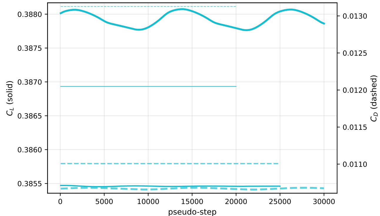
\alpha=2^\circ : C_L , C_D
