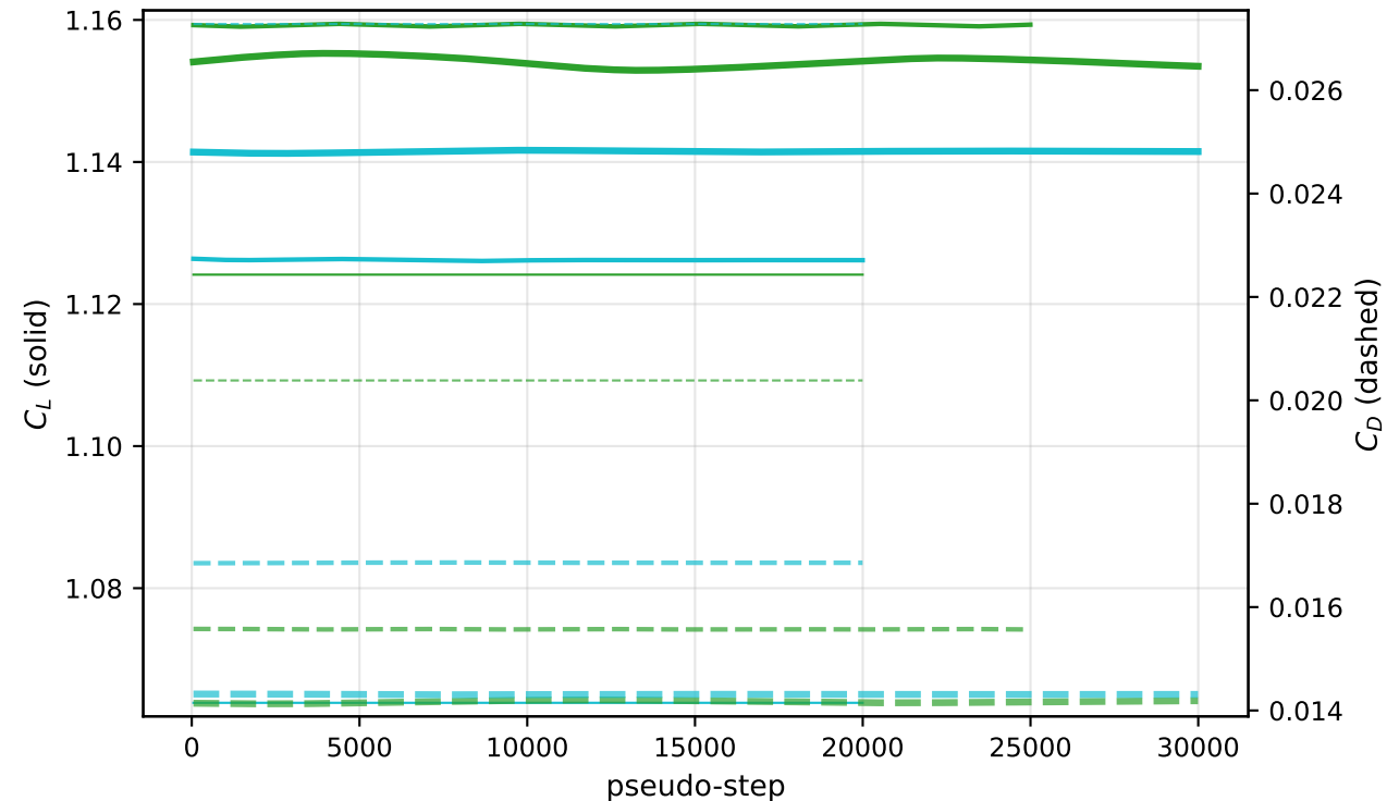
\alpha=8.5^\circ : C_L , C_D
