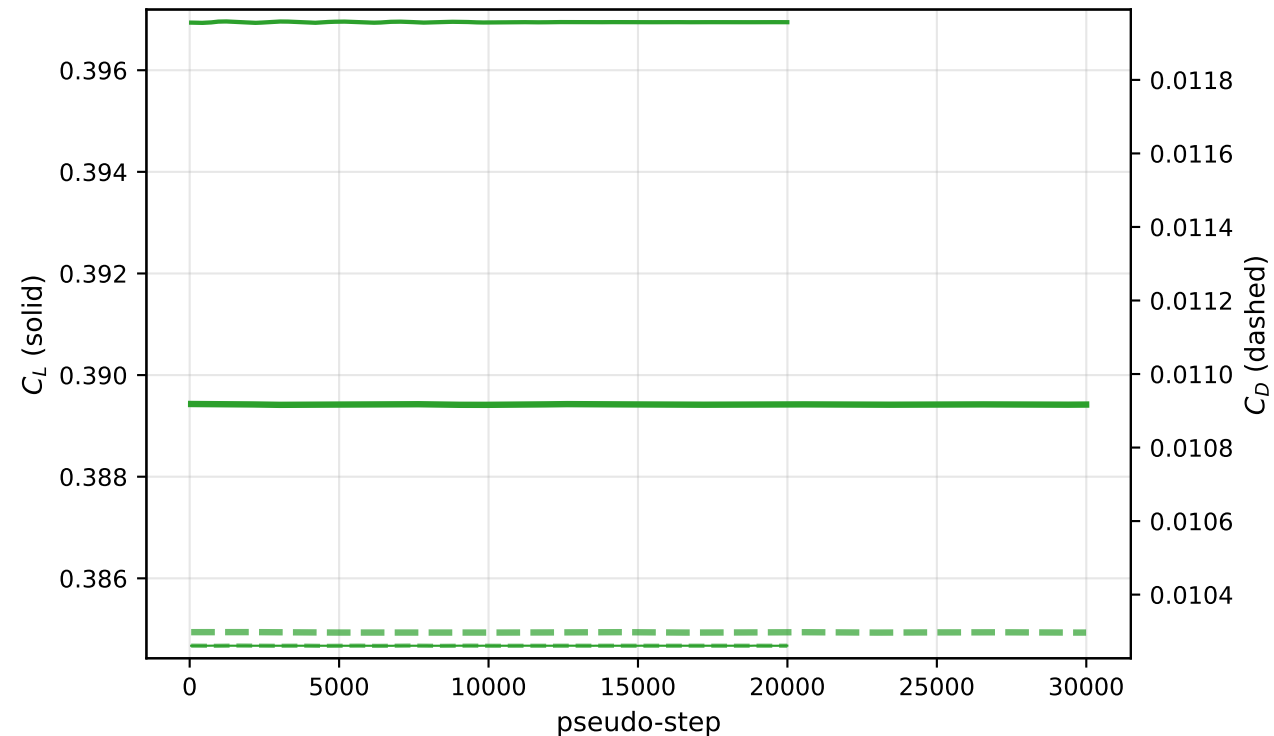
\alpha=5^\circ : C_L , C_D
