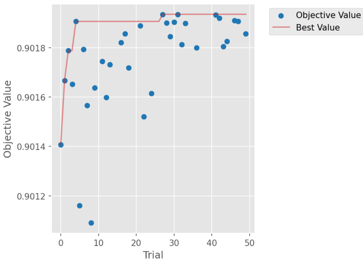
Gambar 4.17 Riwayat optimisasi Optuna pada fine-tuning WavLM+LoRA
