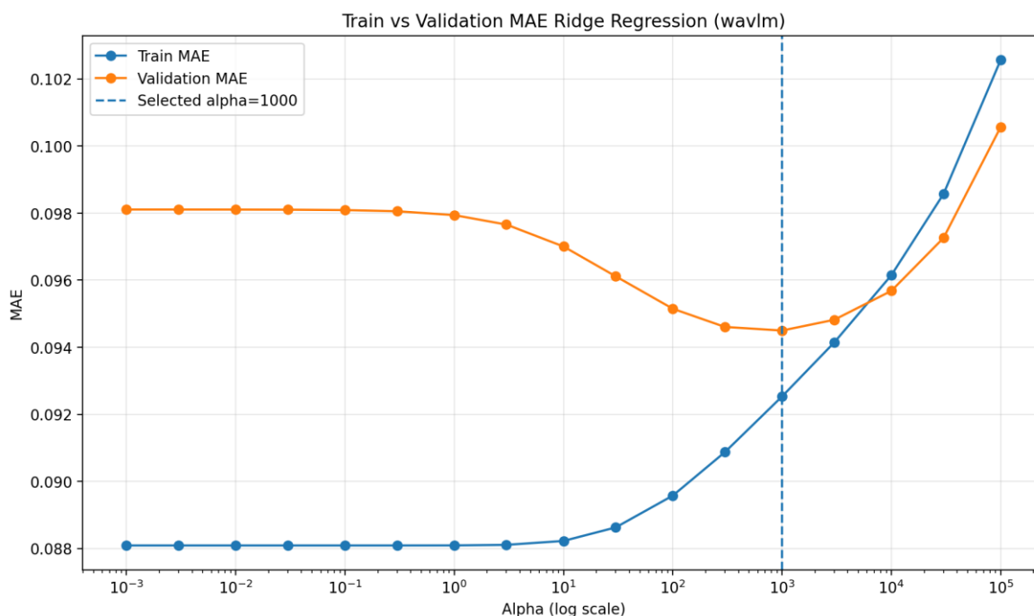
Gambar 4.8 Kurva train MAE dan validation MAE Ridge Regression terhadap nilai alpha pada baseline official split untuk WavLM
