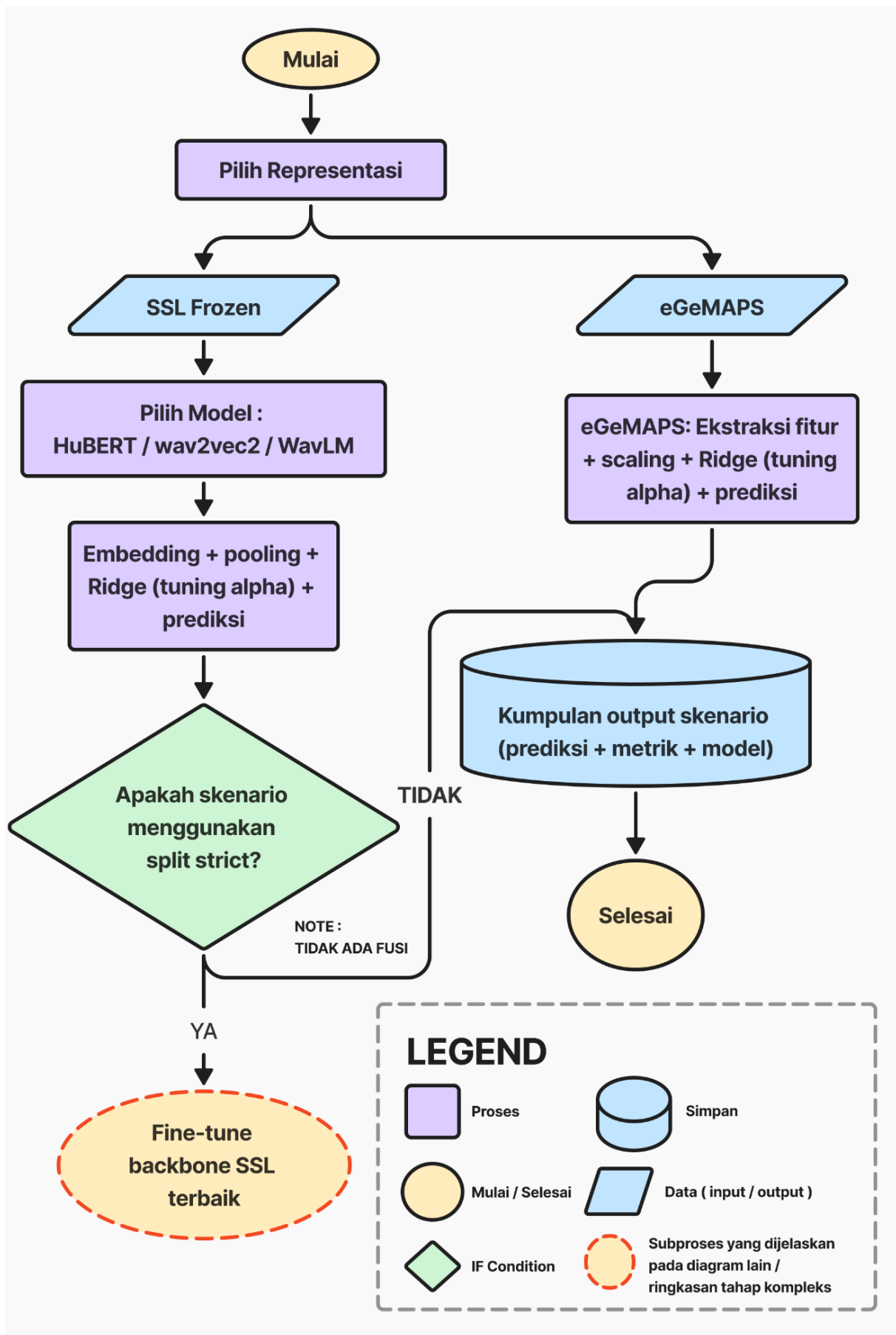
Gambar 3.4 Alur Skenario Baseline dan Representasi Model
