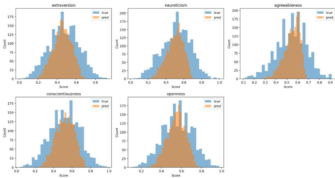
Gambar 4.26 Histogram label aktual dan prediksi HuBERT+LoRA best-val run pada test_strict
