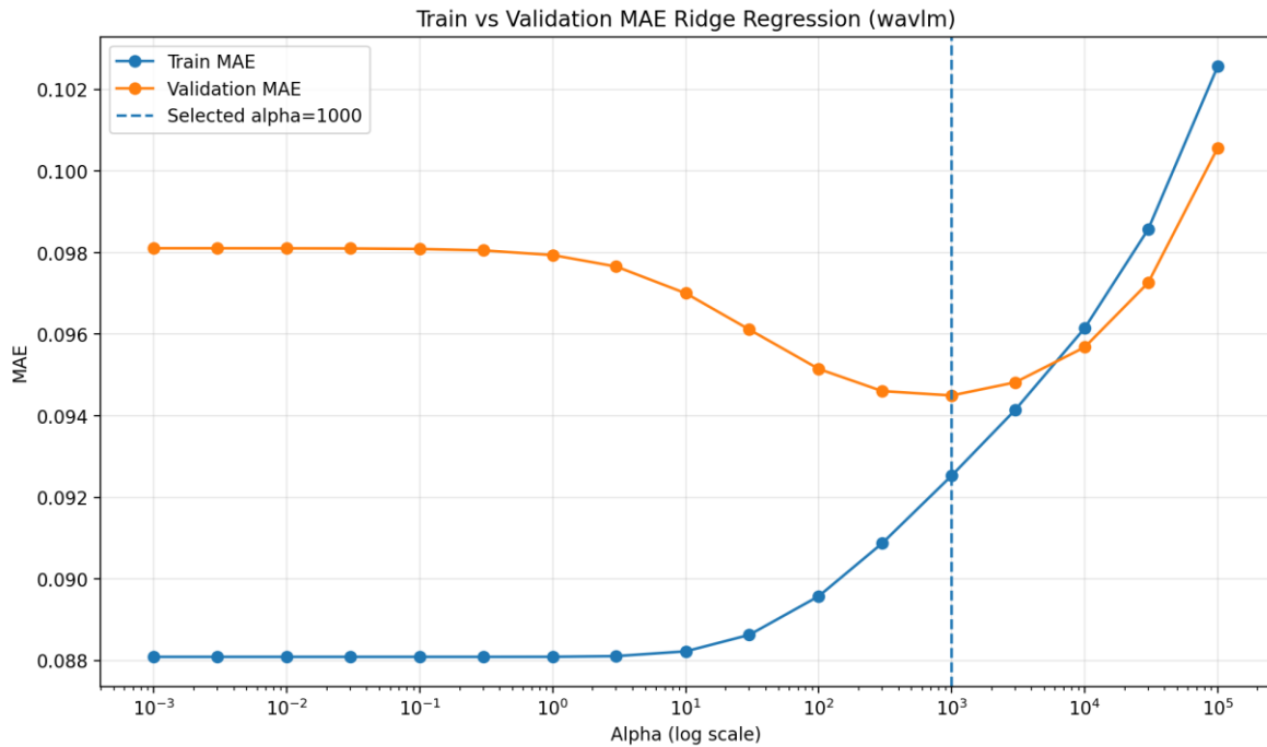
Gambar 4.7 Kurva train MAE dan validation MAE Ridge Regression terhadap nilai alpha pada baseline official split untuk WavLM
