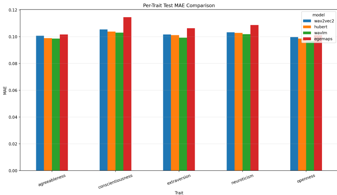
Gambar 4.14 Perbandingan MAE per-trait pada test set strict split
