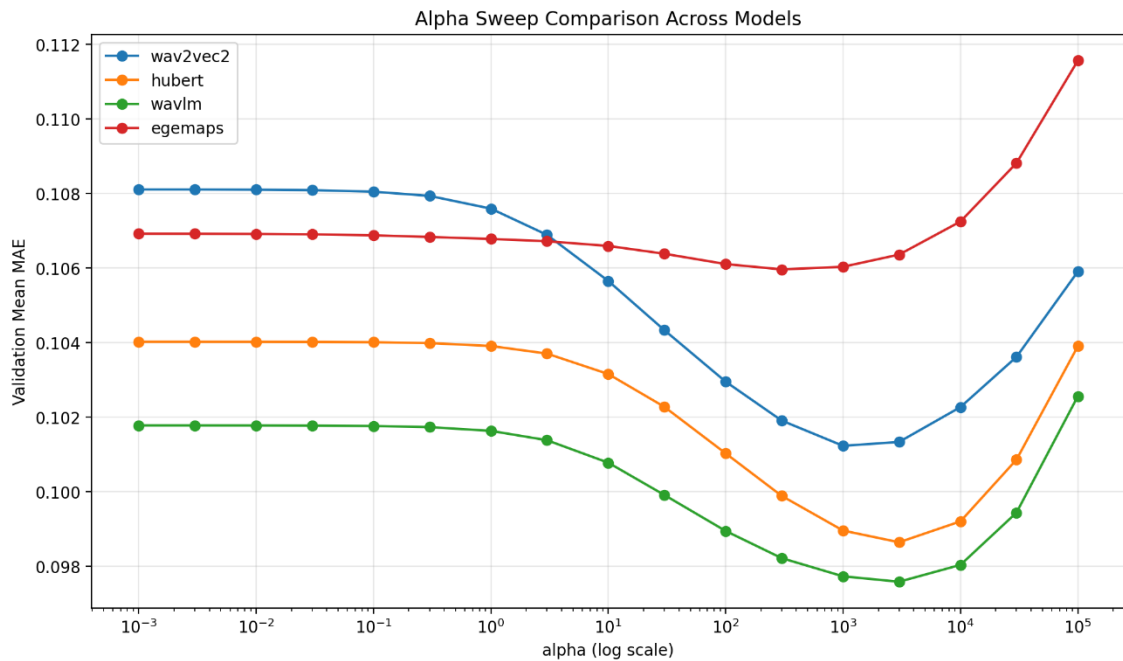
Gambar 4.11 Perbandingan mean MAE validation terhadap nilai alpha pada baseline strict split
