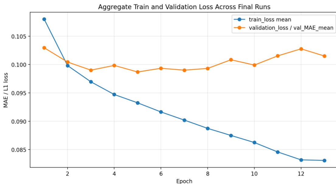
Gambar 4.23 Kurva agregat train loss dan validation loss pada 10 final runs HuBERT+LoRA
