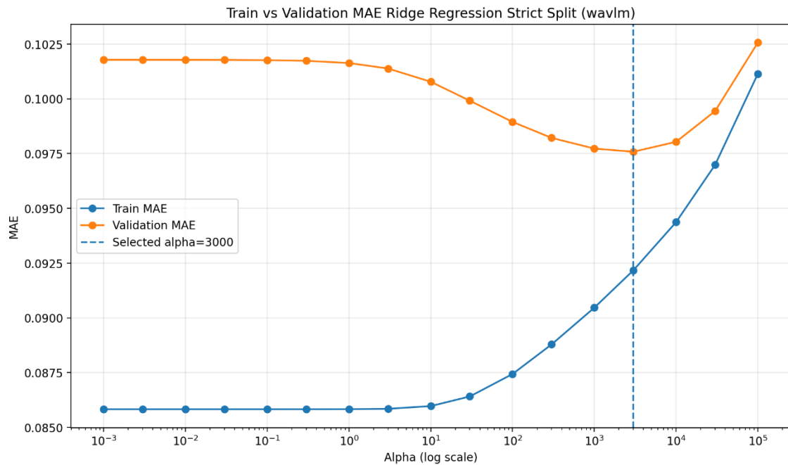
Gambar 4.12 Kurva train MAE dan validation MAE Ridge Regression terhadap alpha pada strict split untuk WavLM
