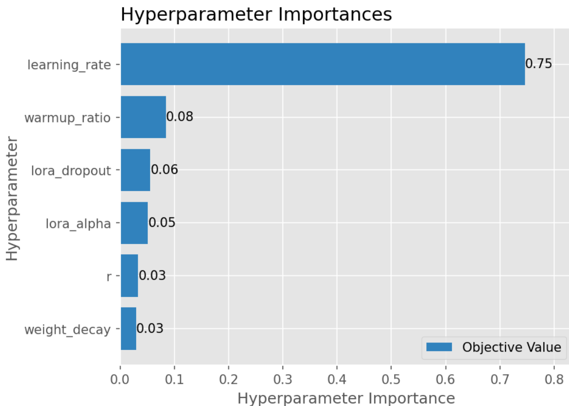
Gambar 4.17 Parameter importance pada studi Optuna WavLM+LoRA
