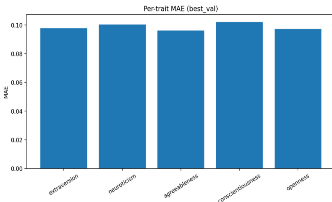
Gambar 4.24 Perbandingan MAE per-trait HuBERT+LoRA best-val run pada test_strict
