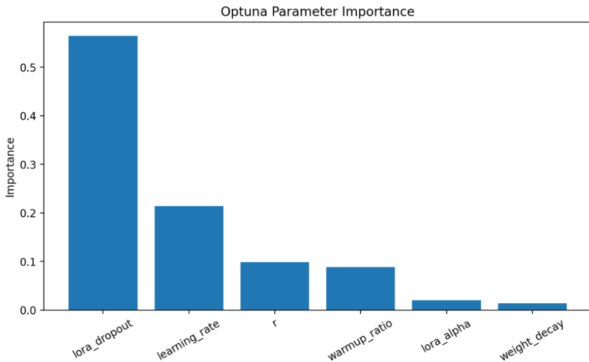
Gambar 4.22 Parameter importance pada studi Optuna HuBERT+LoRA
