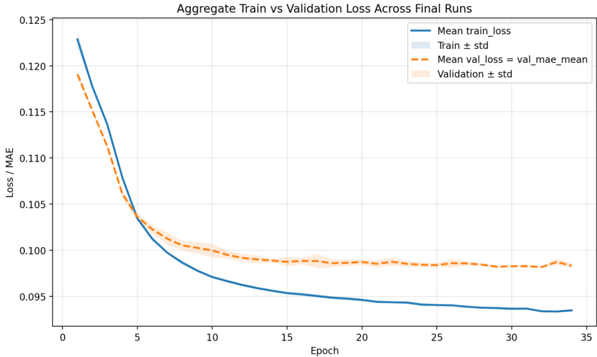
Gambar 4.20 Kurva agregat train loss dan validation loss WavLM+LoRA pada 10 final runs
