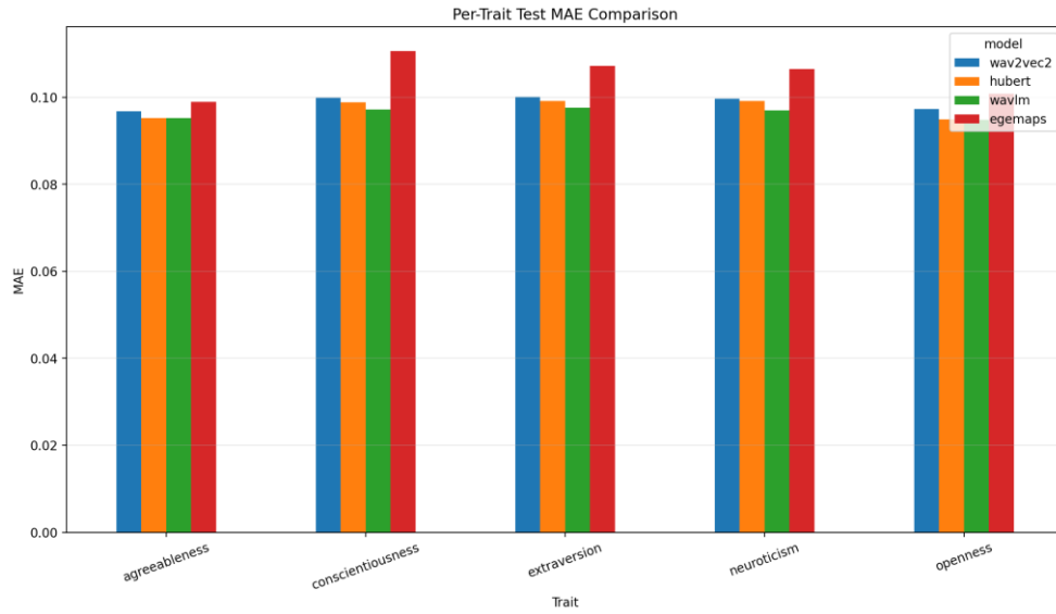
Gambar 4.9 Perbandingan MAE per-trait pada test set official split
