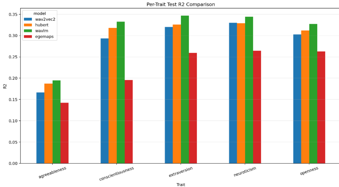
Gambar 4.15 Perbandingan R^2 per-trait pada test set strict split
