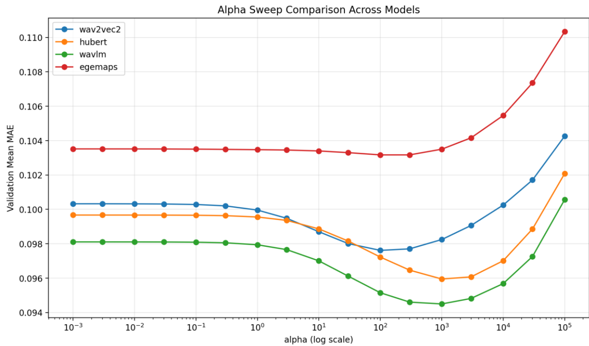
Gambar 4.6 Perbandingan mean MAE validation terhadap nilai alpha pada baseline official split
