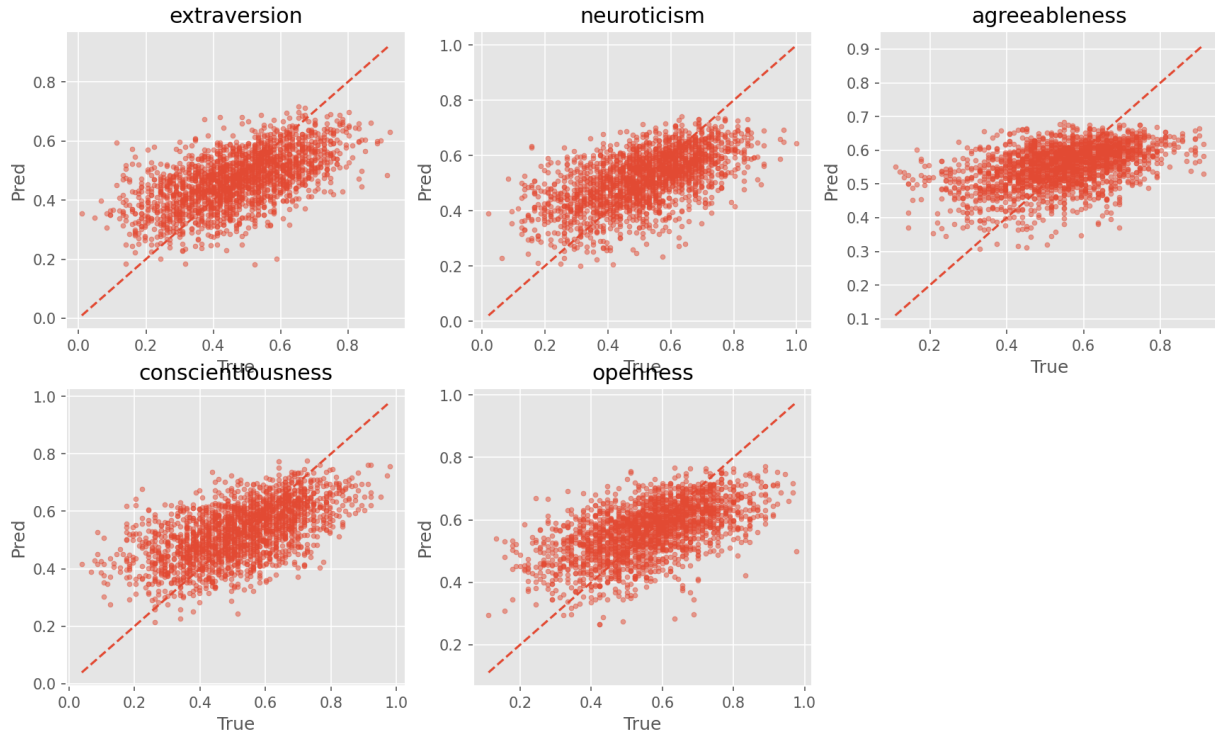
Gambar 4.19 Scatter plot label aktual dan prediksi WavLM+LoRA best-val run pada test_strict
