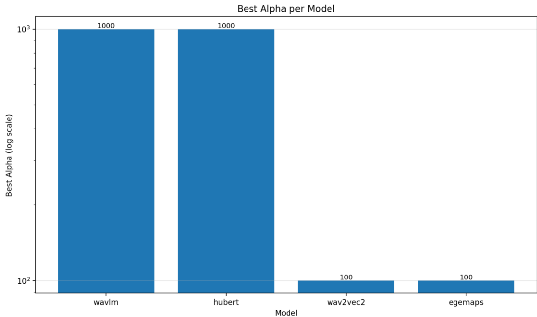
Lampiran 16 Grafik best alpha per metode pada baseline official split
