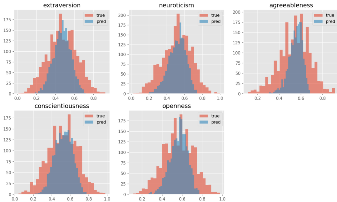
Gambar 4.18 Histogram label aktual dan prediksi WavLM+LoRA best-val run pada test_strict
