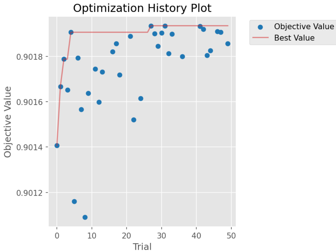
Gambar 4.16 Riwayat optimisasi Optuna pada fine-tuning WavLM+LoRA
