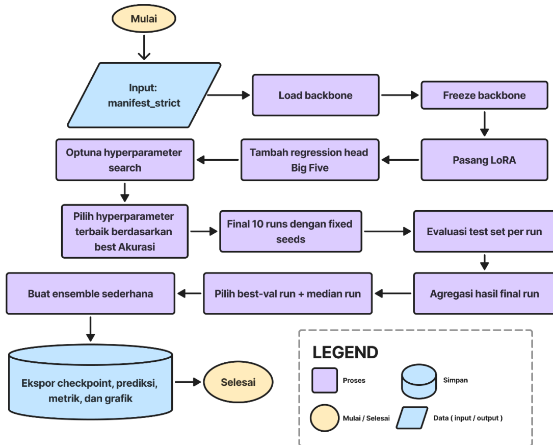
Gambar 3.5 Diagram Alir Strategi Fine-tuning dengan LoRA
