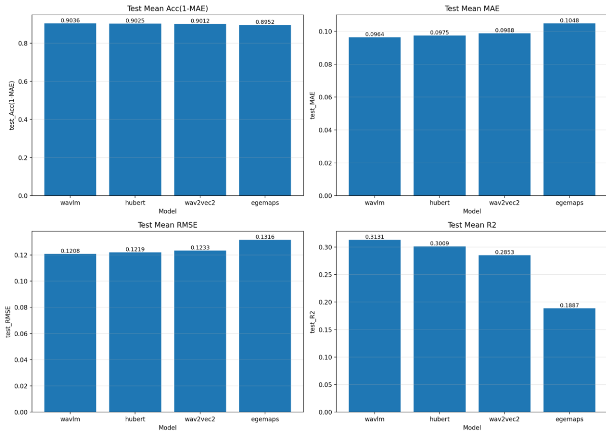
Gambar 4.8 Perbandingan metrik rata-rata antar metode pada test set official split
