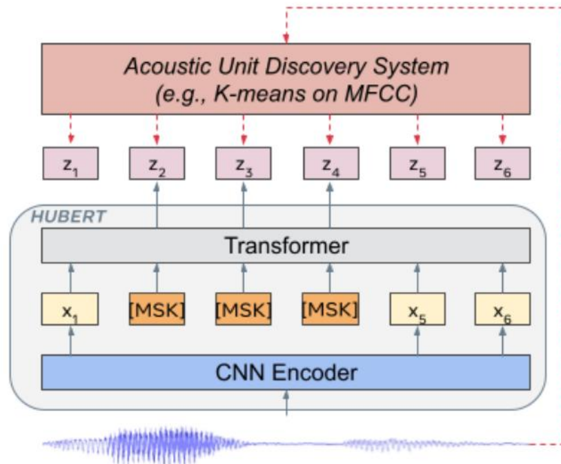
Gambar 2.3 Skema HuBERT untuk memprediksi assignment cluster pada frame yang dilakukan masking (Hsu dkk., 2021).
