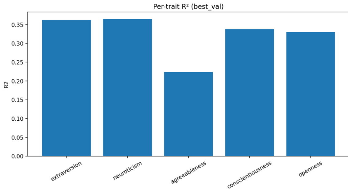
Gambar 4.25 Perbandingan R^2 per-trait HuBERT+LoRA best-val run pada test_strict
