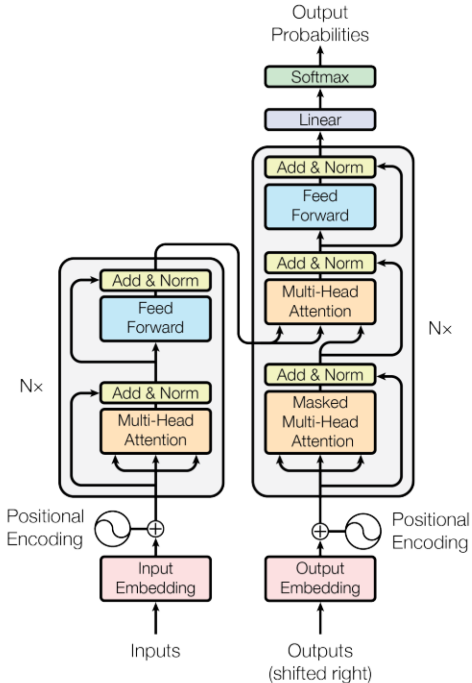
Gambar 2.1 Arsitektur Transformer (Vaswani dkk., 2017)
