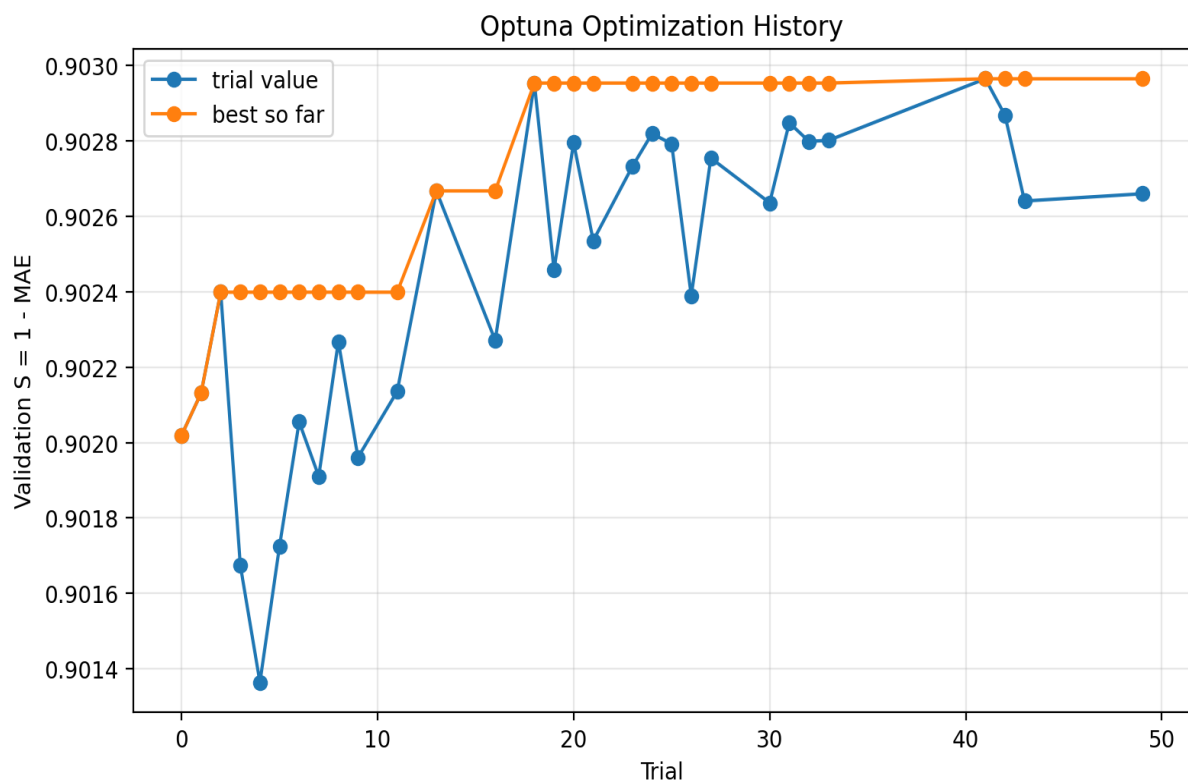
Gambar 4.21 Riwayat optimisasi Optuna pada fine-tuning HuBERT+LoRA
