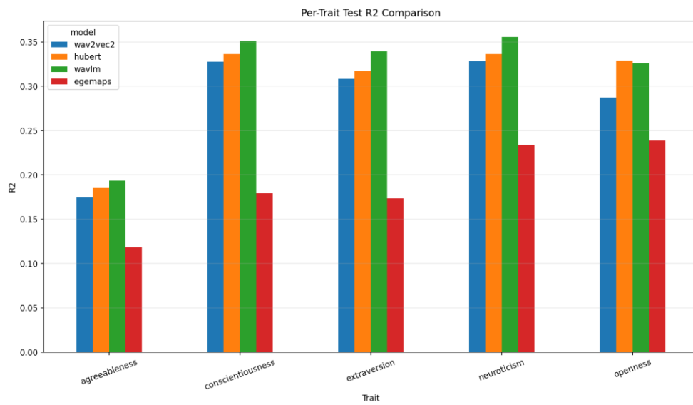
Gambar 4.10 Perbandingan R^2 per-trait pada test set official split
