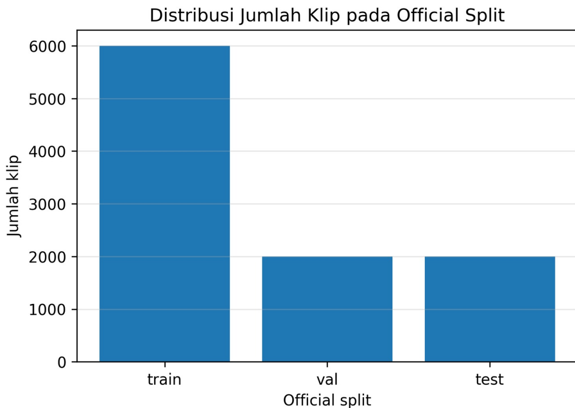
Gambar 4.1 Distribusi official split awal pada dataset.
