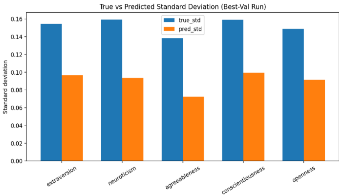
Gambar 4.28 Perbandingan simpangan baku label aktual dan prediksi HuBERT+LoRA best-val run pada test_strict .
