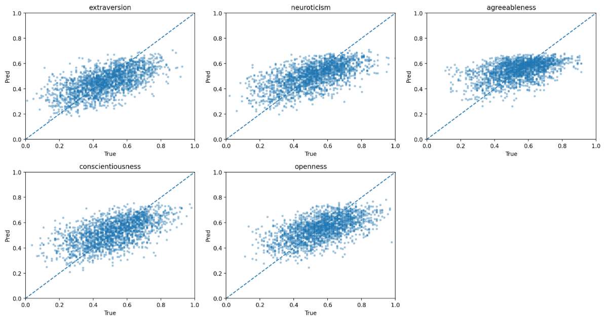
Gambar 4.27 Scatter plot label aktual dan prediksi HuBERT+LoRA best-val run pada test_strict
