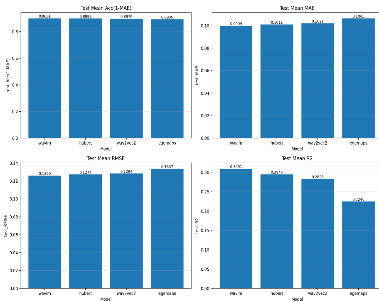
Gambar 4.13 Perbandingan metrik rata-rata antar metode pada test set strict split
