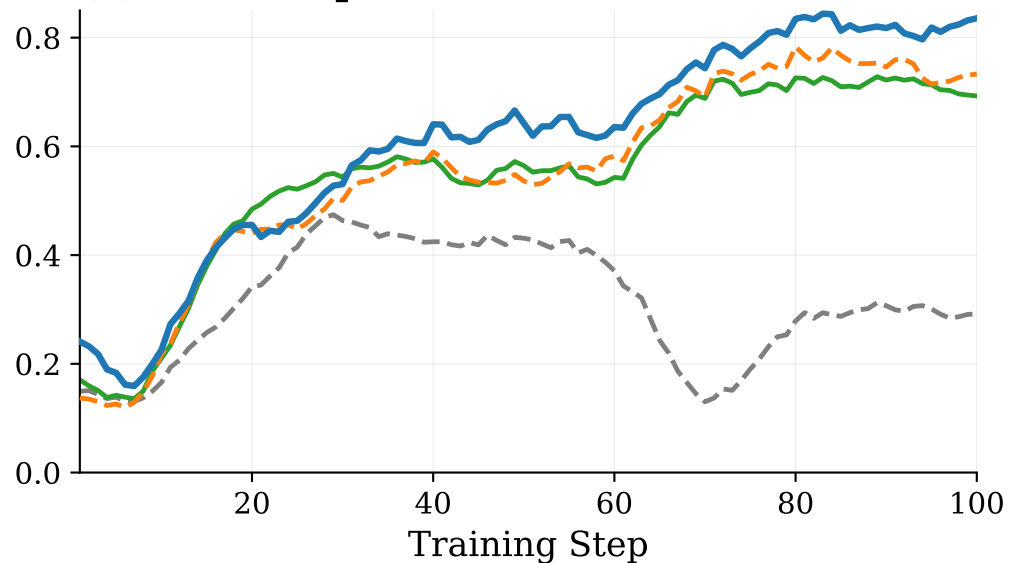
(d) WebShop 3B
