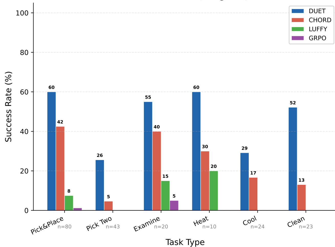
ALFWorld 1.5B (val@100)
