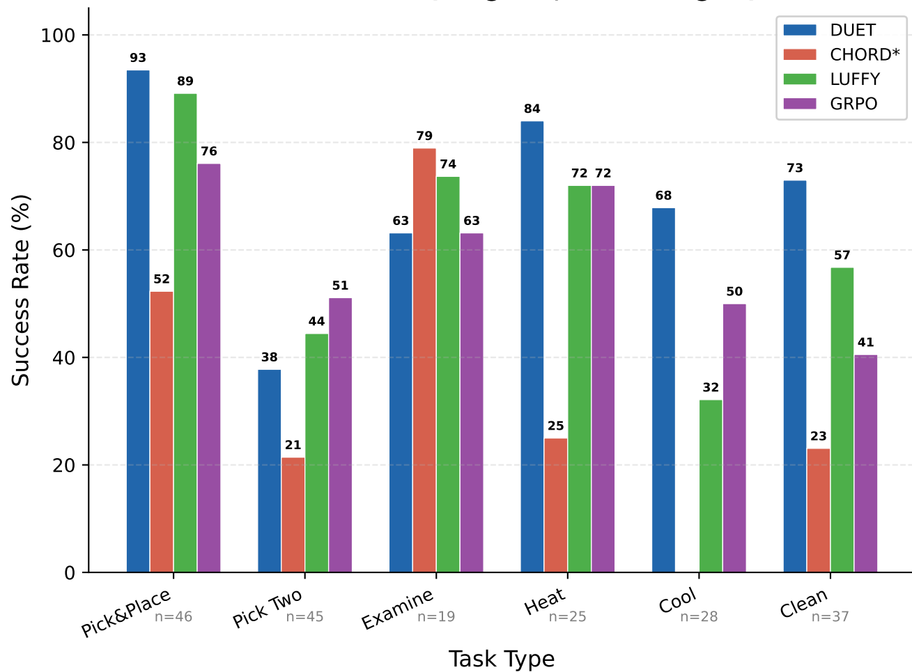
ALFWorld 3B (val@100, CHORD* @50)
