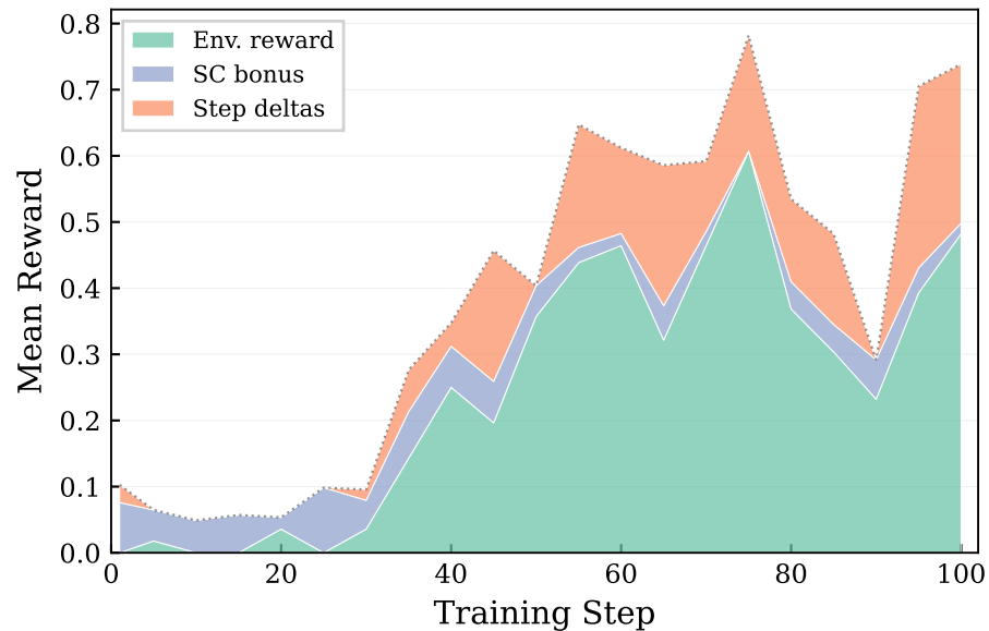
ALFWorld — Qwen2.5-1.5B
