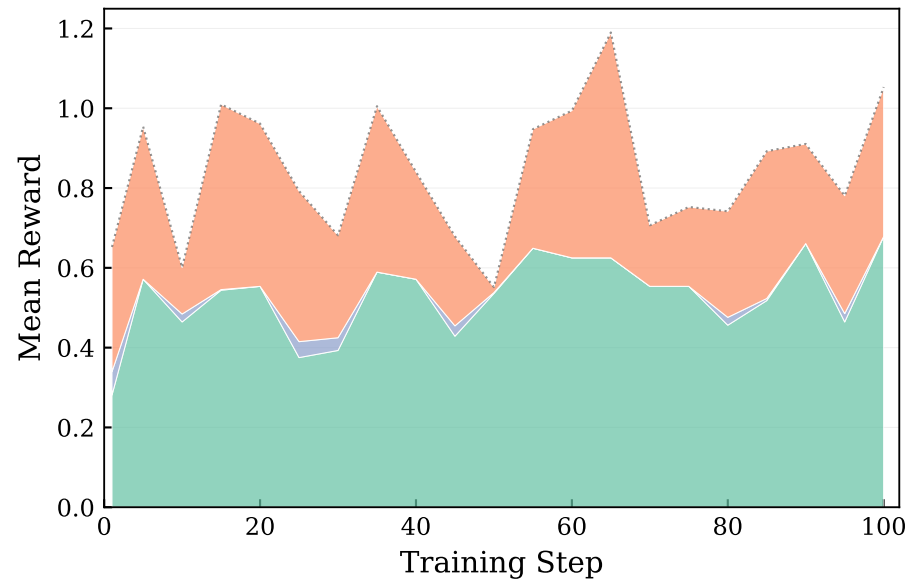
ALFWorld — Qwen2.5-3B
