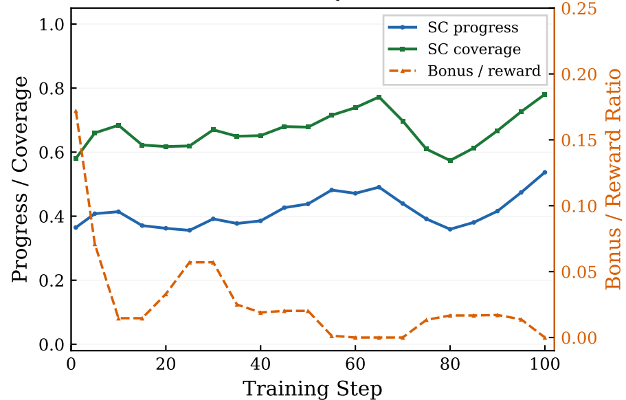
ALFWorld — Qwen2.5-3B
