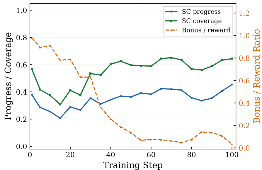
ALFWorld — Qwen2.5-1.5B
