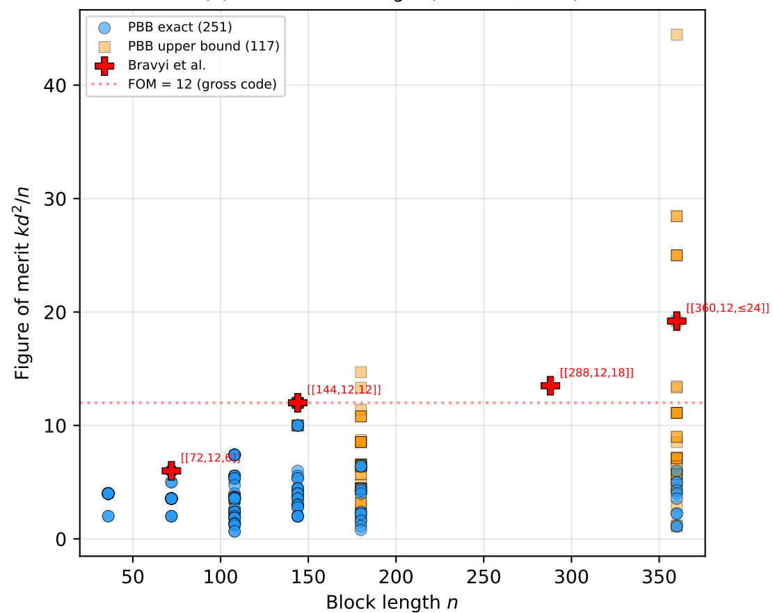
(d) FOM vs block length (non-CSS, d \geq 6 )
