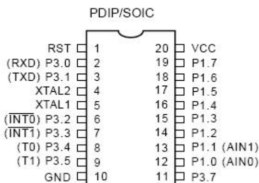
图 4-9 2051 信号引脚图
