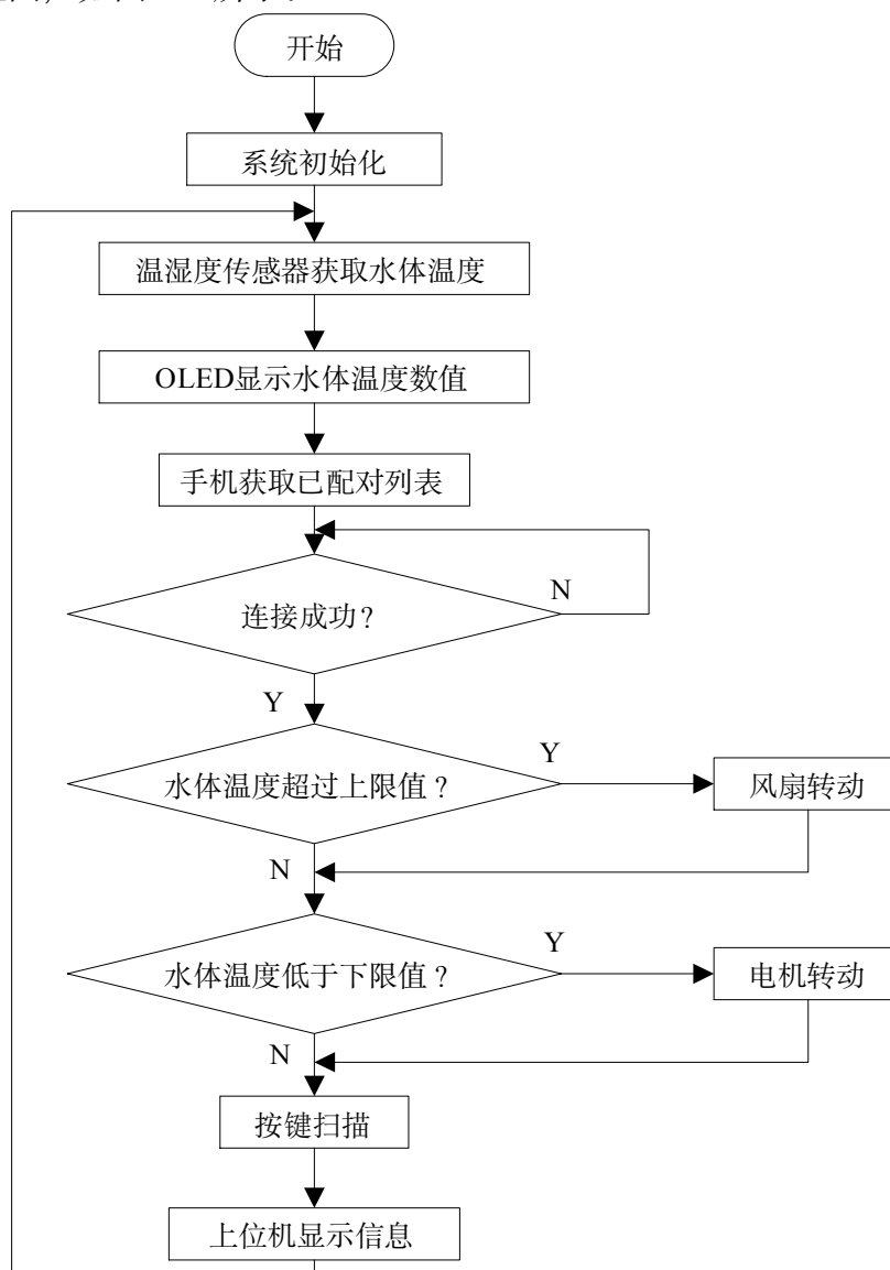
图 5-1 系统流程图
