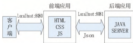
图1 前后端分离开发模式
