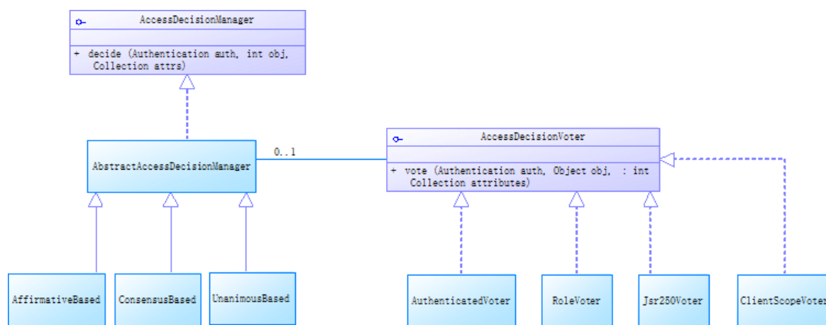
图 2.9 Spring Security 访问决策管理器源码解读
