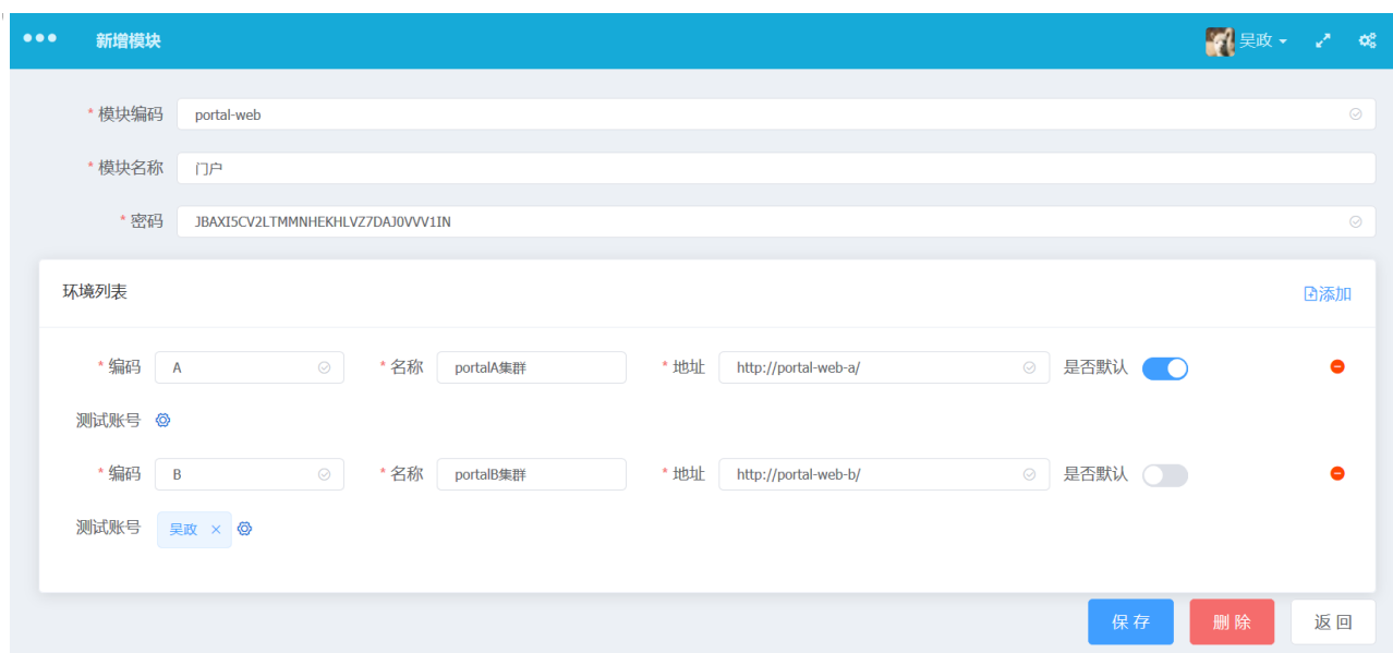
图 4.29 前端模块环境切换配置
