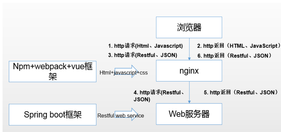
图 2.19 基于 Vue 的前后端彻底分离的部署模式
