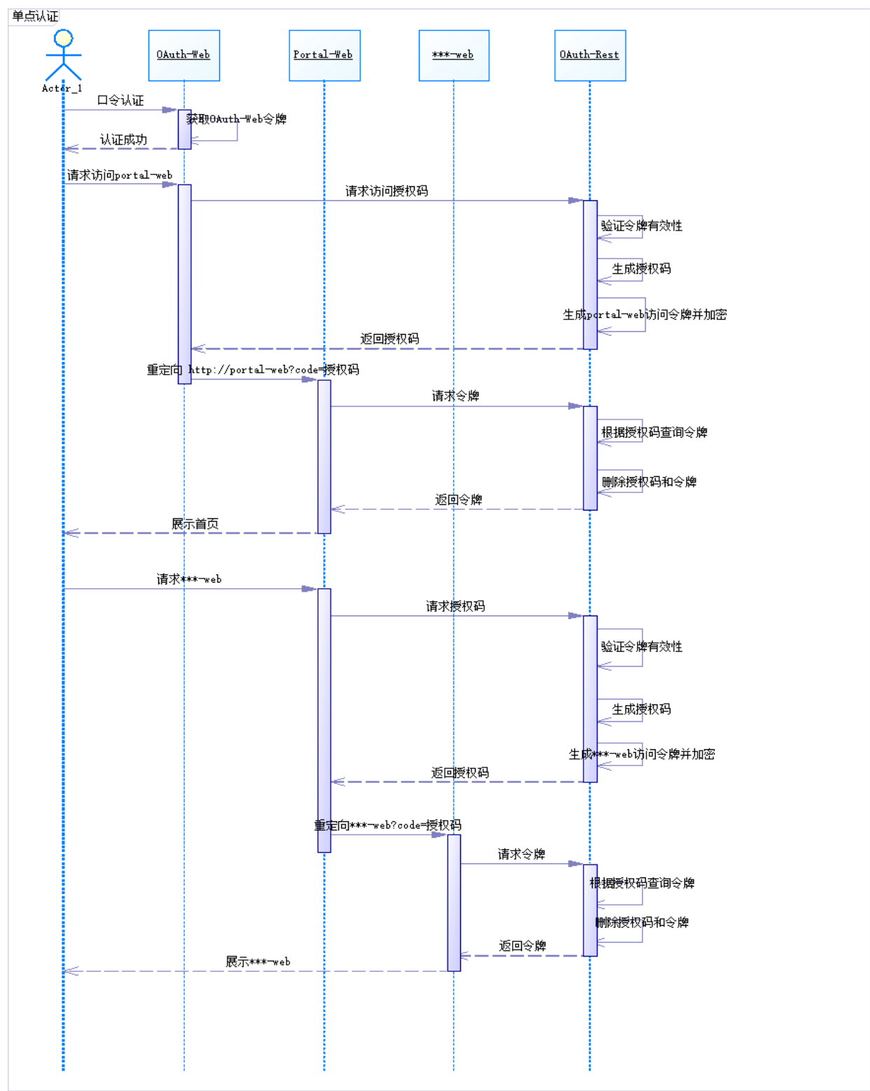
图 3.9 单点认证流程
