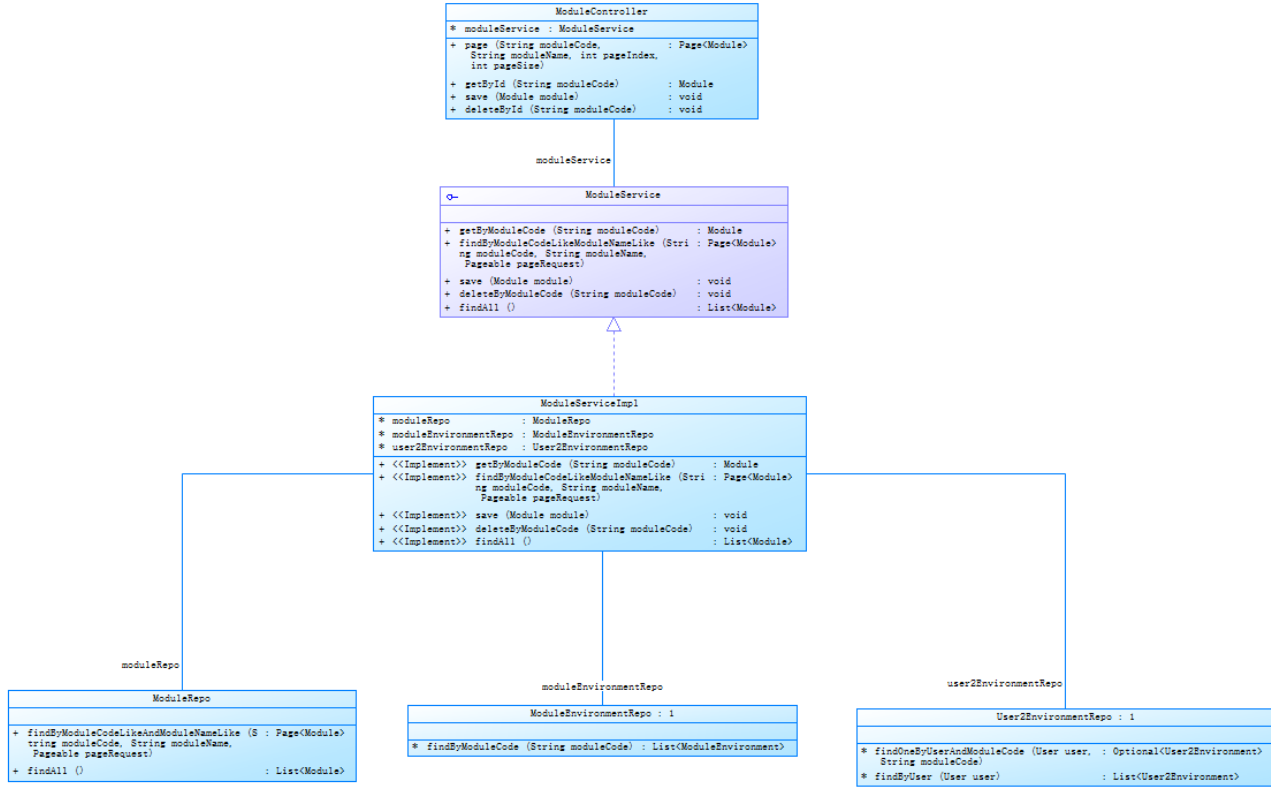
图 4.19 模块管理功能实现
