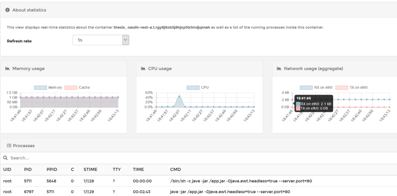
图 4.25 容器性能监控
