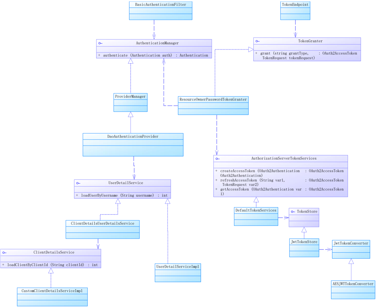
图 4.13 基于 spring oauth2.0 口令认证
