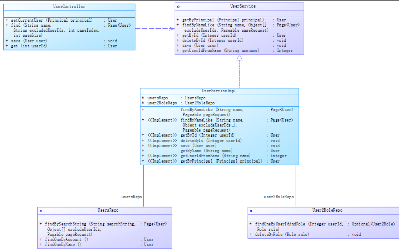
图 4.16 用户管理功能实现
