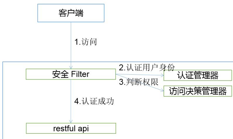
图 2.7 Spring Security 工作原理
