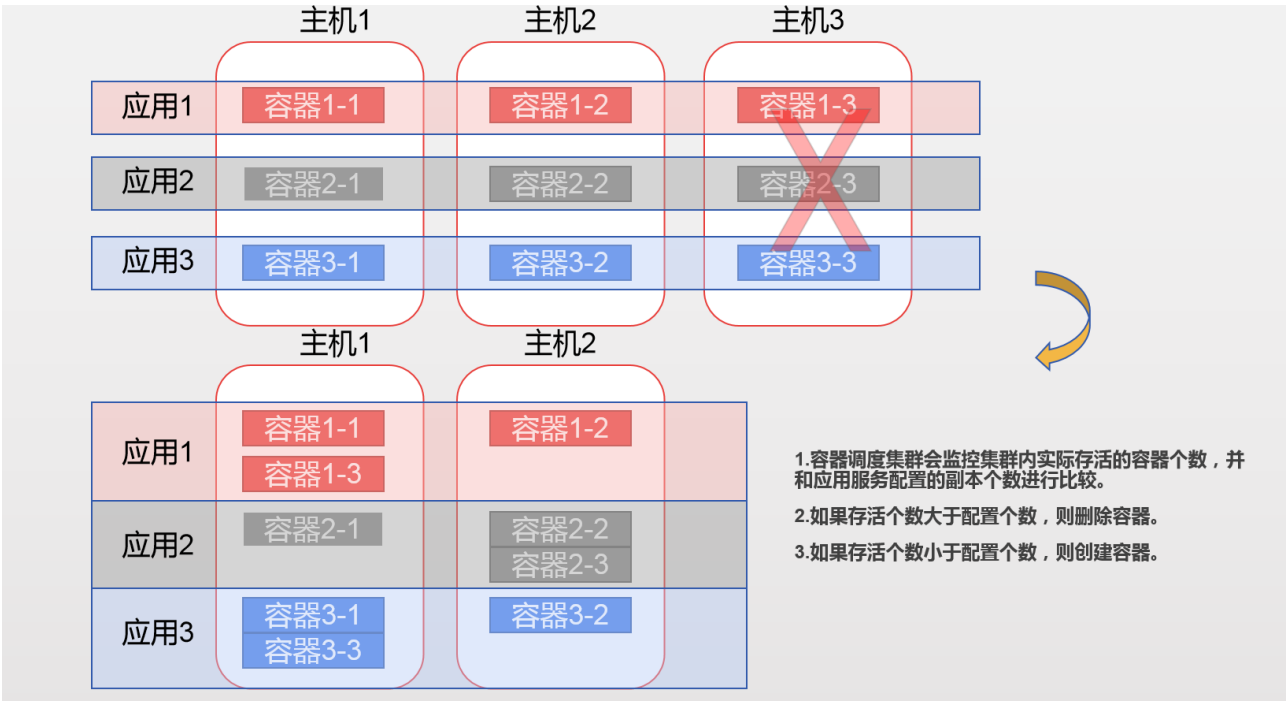
图 2.22 基于 docker swarm service 的容灾方案
