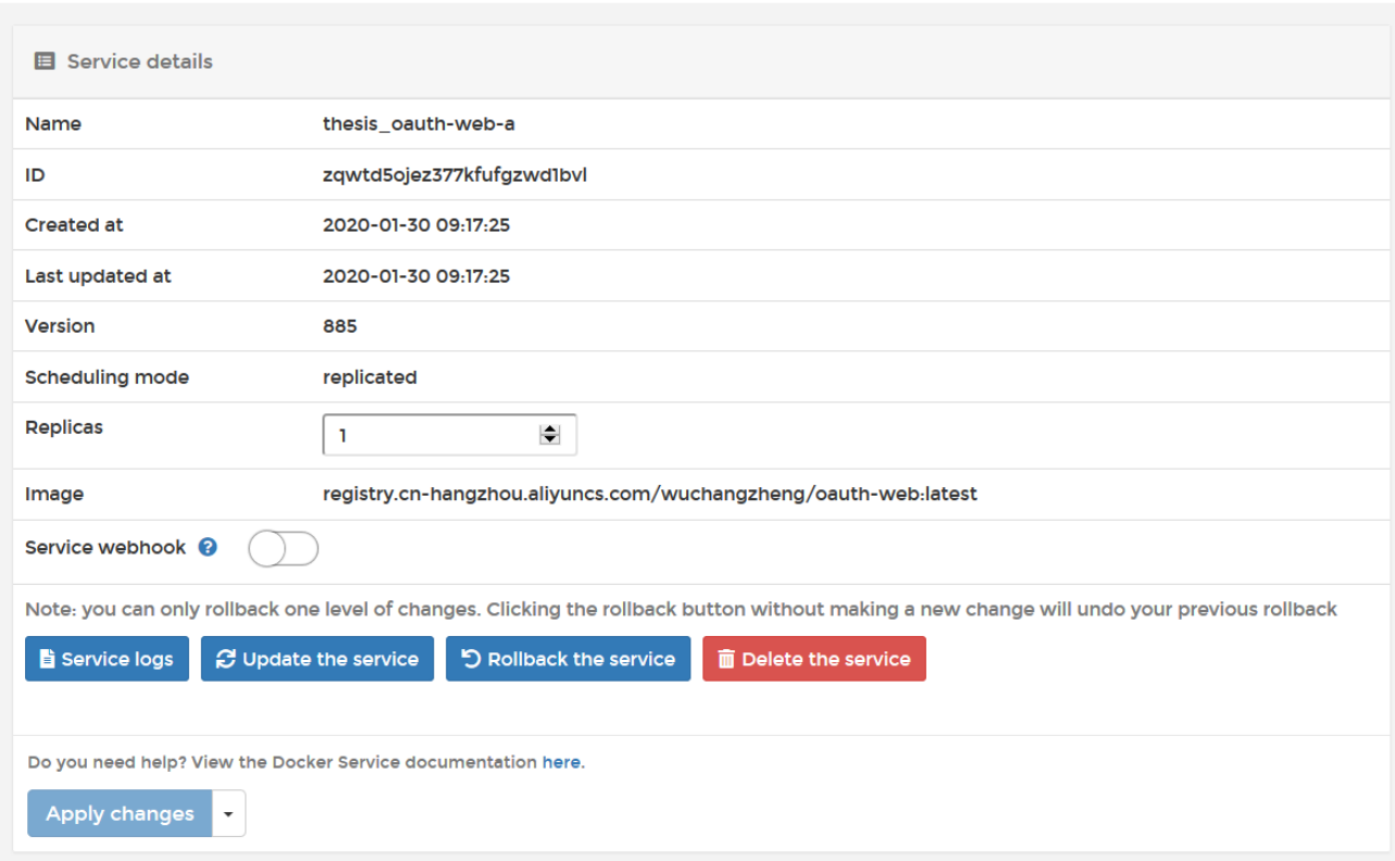
图 4.24 服务详情页面
