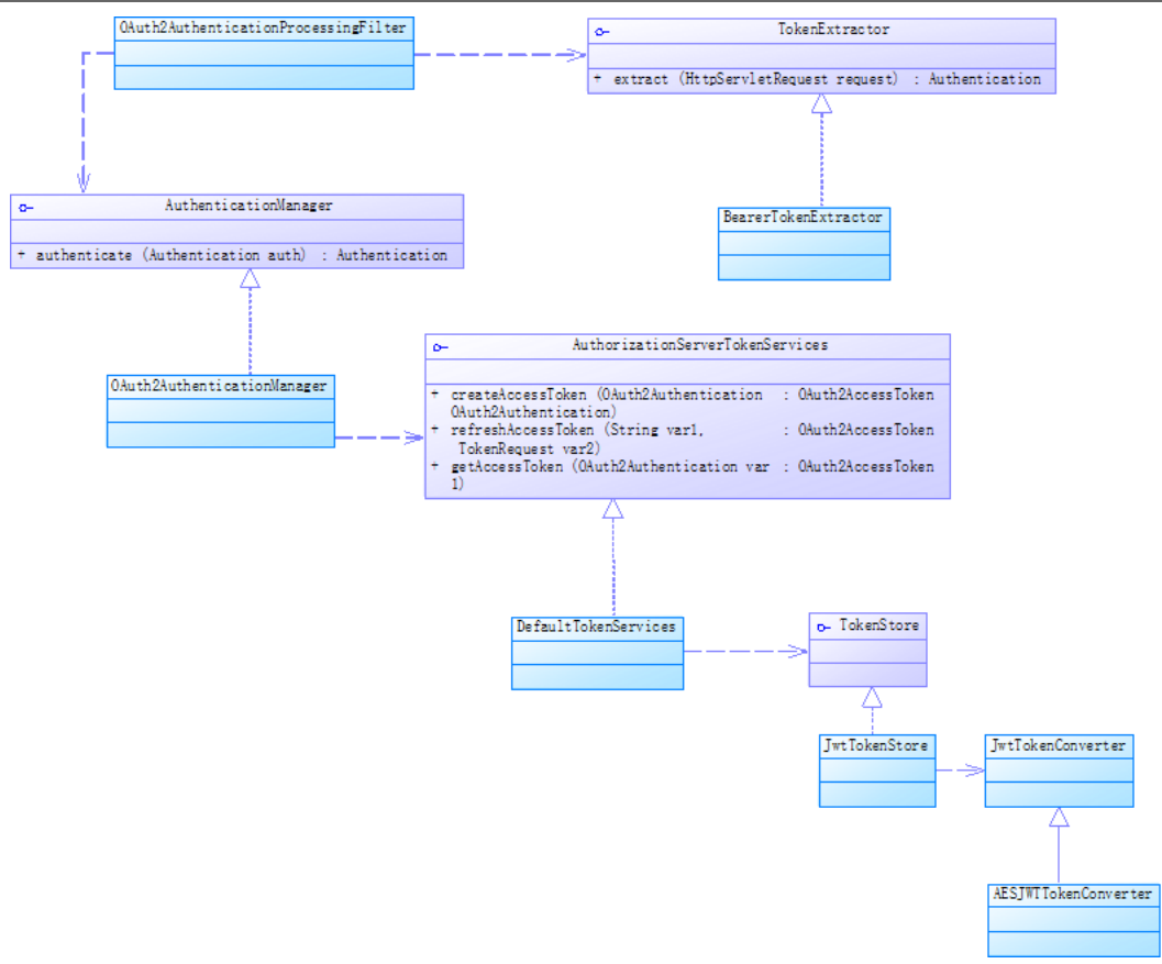
图 4.15 基于 spring oauth2.0 令牌认证
