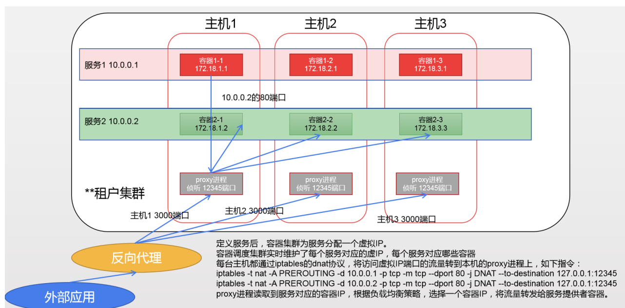
图 2.21 基于 docker swarm service 实现 web 服务的负载均衡
