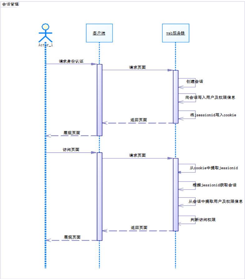
图 2.13 web 服务会话管理
