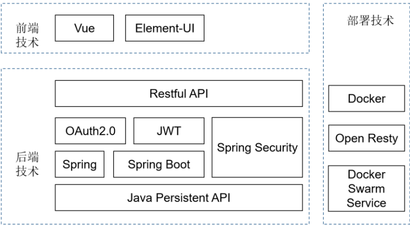
图 3.3 系统技术架构
