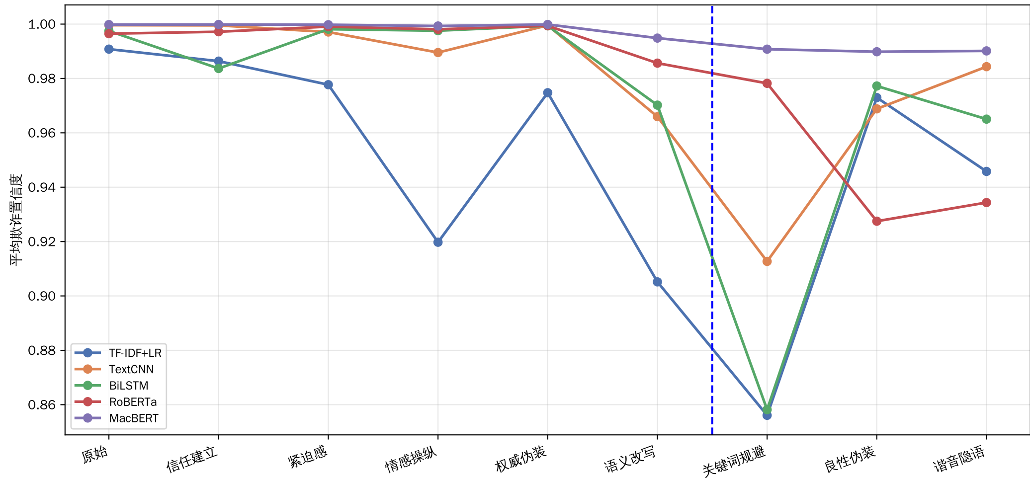
各模型对欺诈样本的平均预测置信度随改写策略的变化
