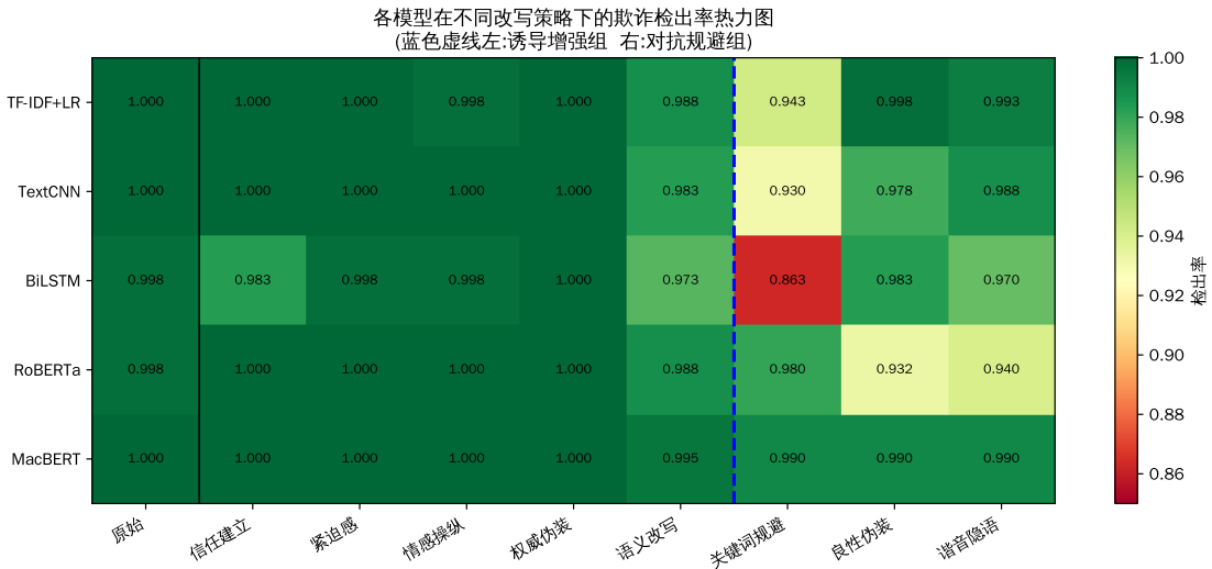
图 6: 各模型在不同改写策略下的欺诈检出率热力图。蓝色虚线左侧为诱导增强组, 右侧为对抗规避组。颜色越绿表示检出率越高 (越鲁棒), 越红表示越脆弱。
