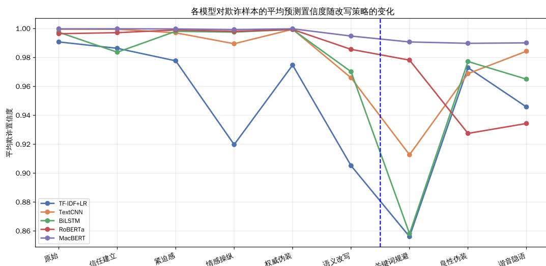
图 8: 各模型对欺诈样本的平均预测置信度随改写策略的变化。预训练模型曲线平稳, 浅层模型在对抗规避组置信度明显下滑。
