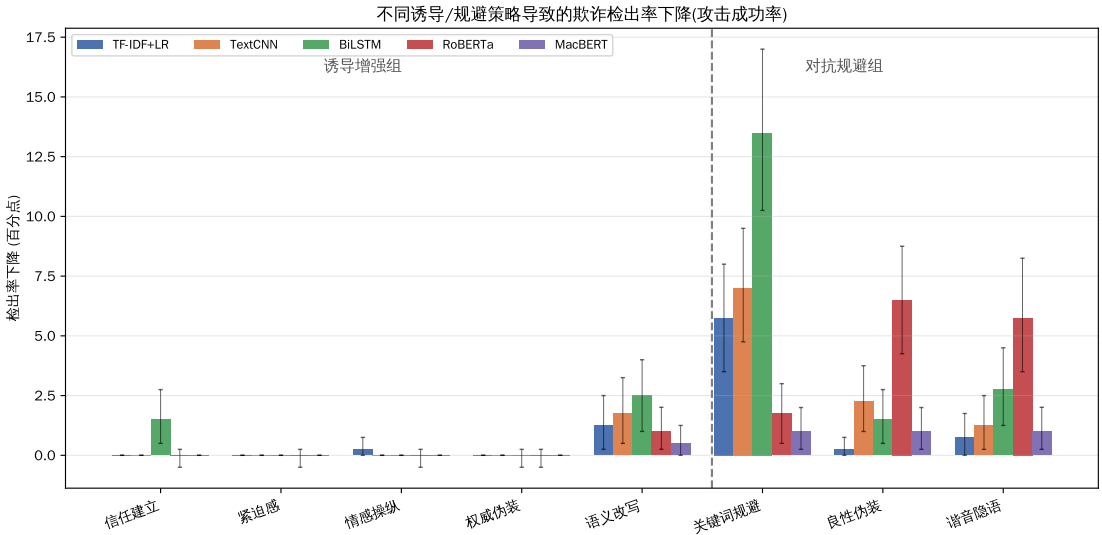
图 7: 不同策略导致的欺诈检出率下降 (攻击成功率)。诱导增强组几乎不造成下降, 对抗规避组 (尤其关键词规避) 造成显著下降。
