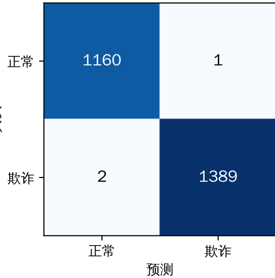
RoBERTa
