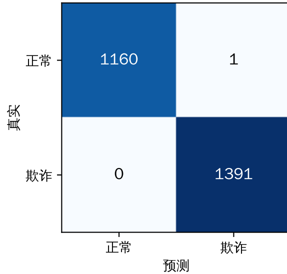
MacBERT
