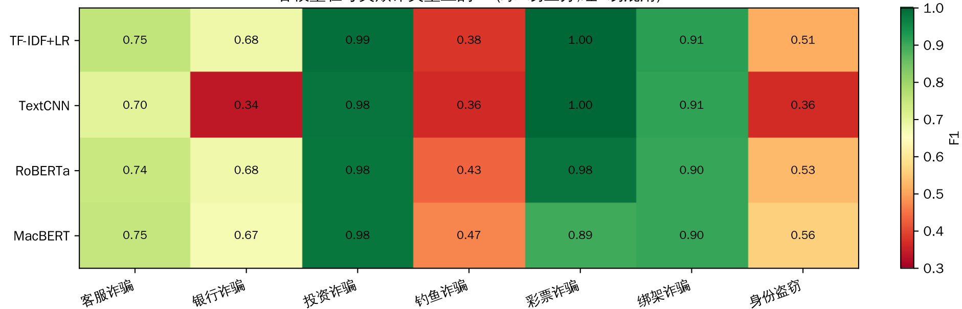
各模型在每类欺诈类型上的 F1(绿=易区分,红=易混淆)
