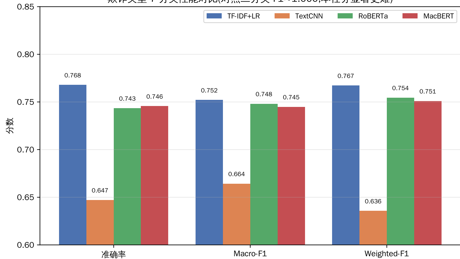
欺诈类型 7 分类性能对比(对照二分类 F1 \approx 1.000,本任务显著更难)
