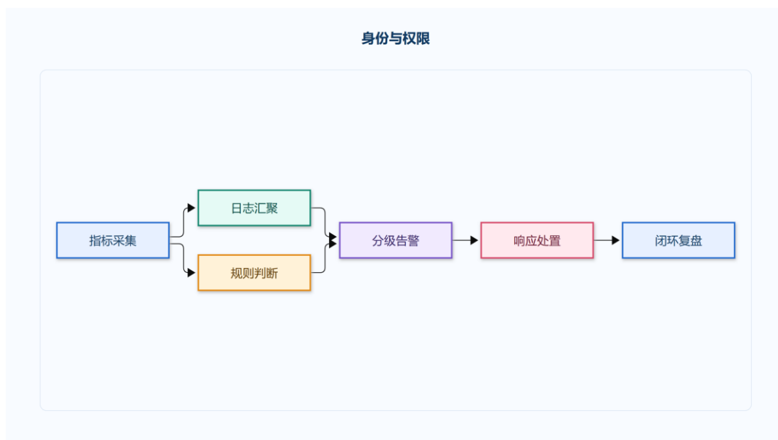
图 5.2 身份与权限
