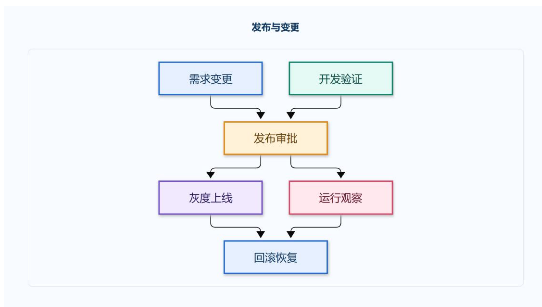
图 5.3 发布与变更
