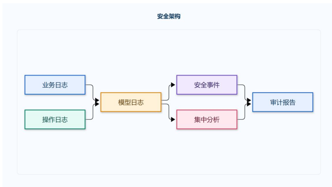
图 4.2 安全架构
