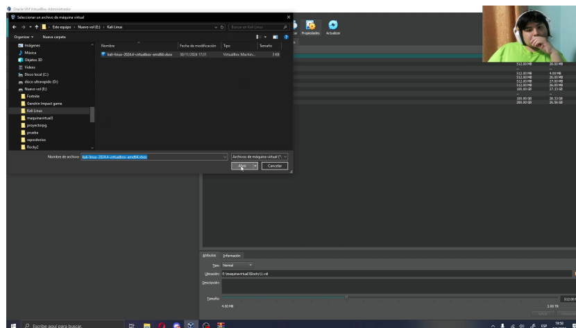
Рис. 2.5: файл VM
