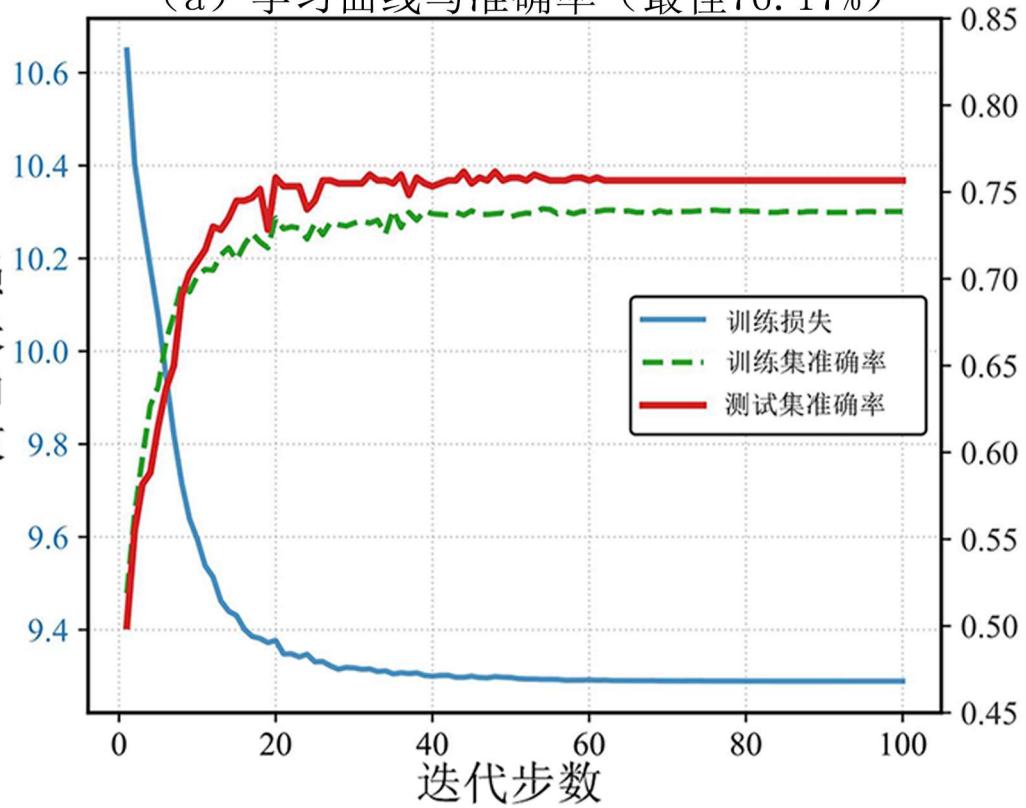
(a) 学习曲线与准确率 (最佳76.17%)
