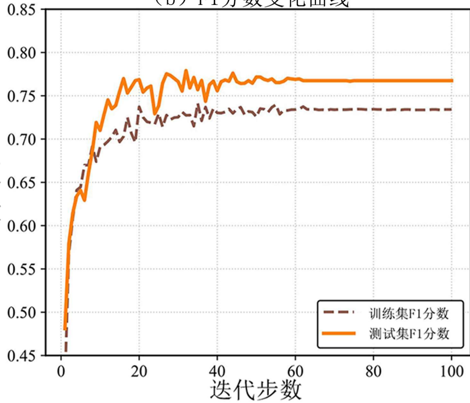
(b) F1分数变化曲线
