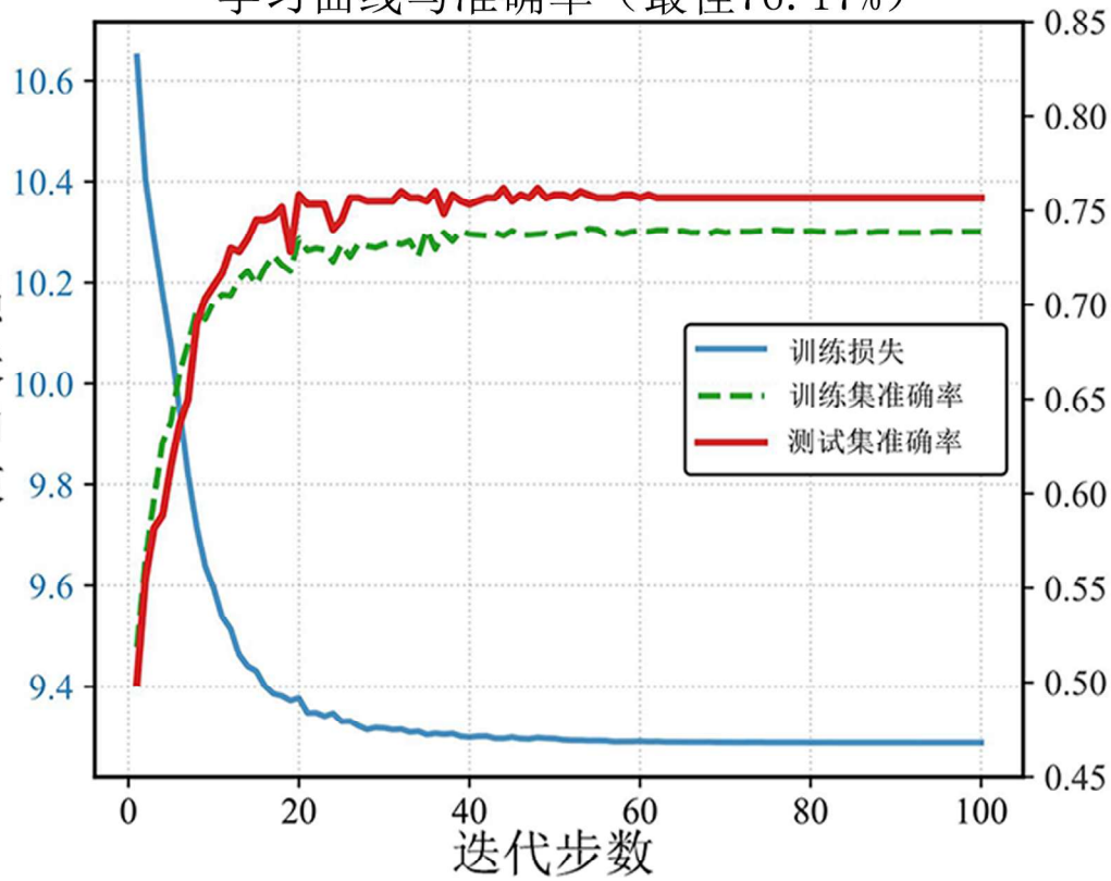
学习曲线与准确率（最佳76.17%）
