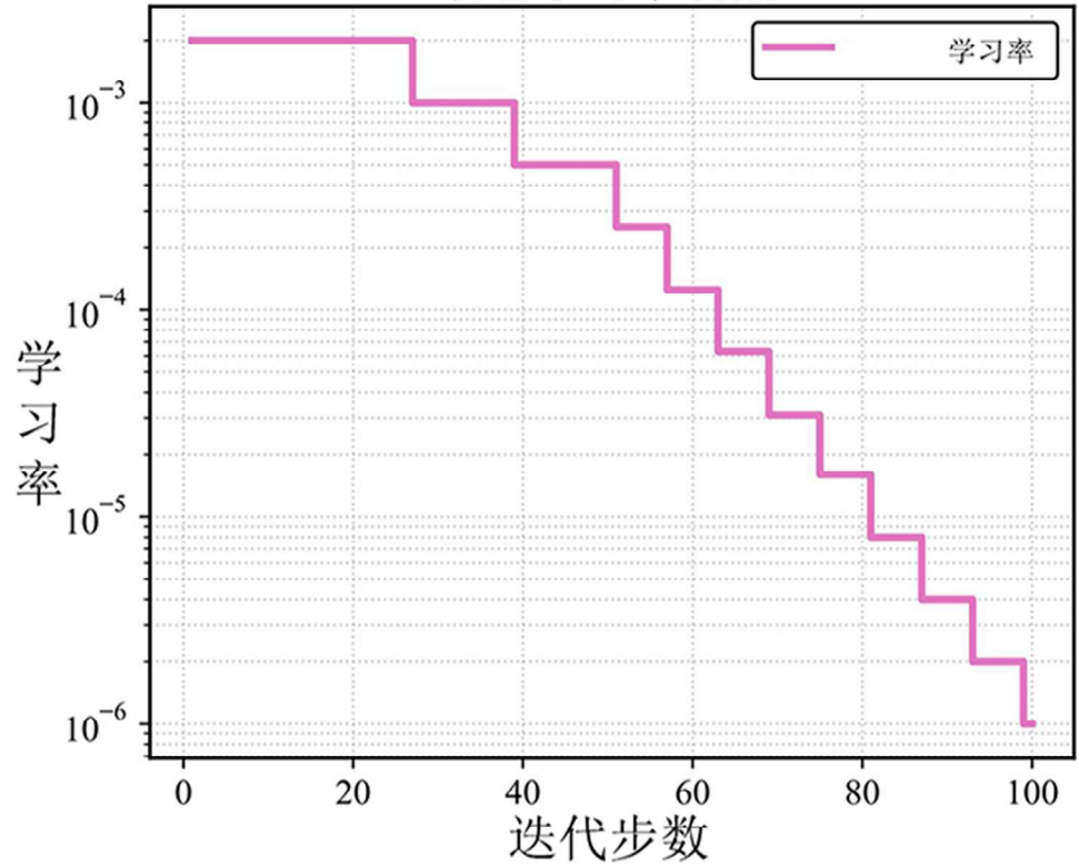
动态学习率衰减
