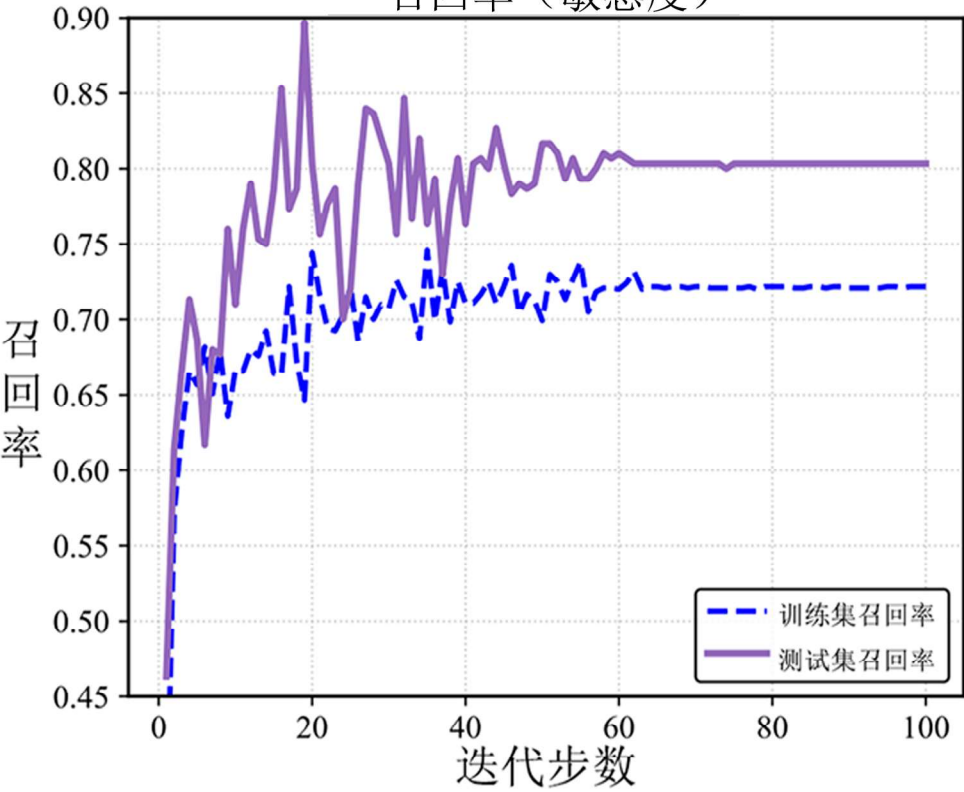
召回率（敏感度）
