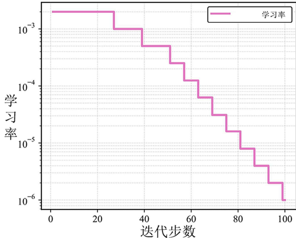
动态学习率衰减
