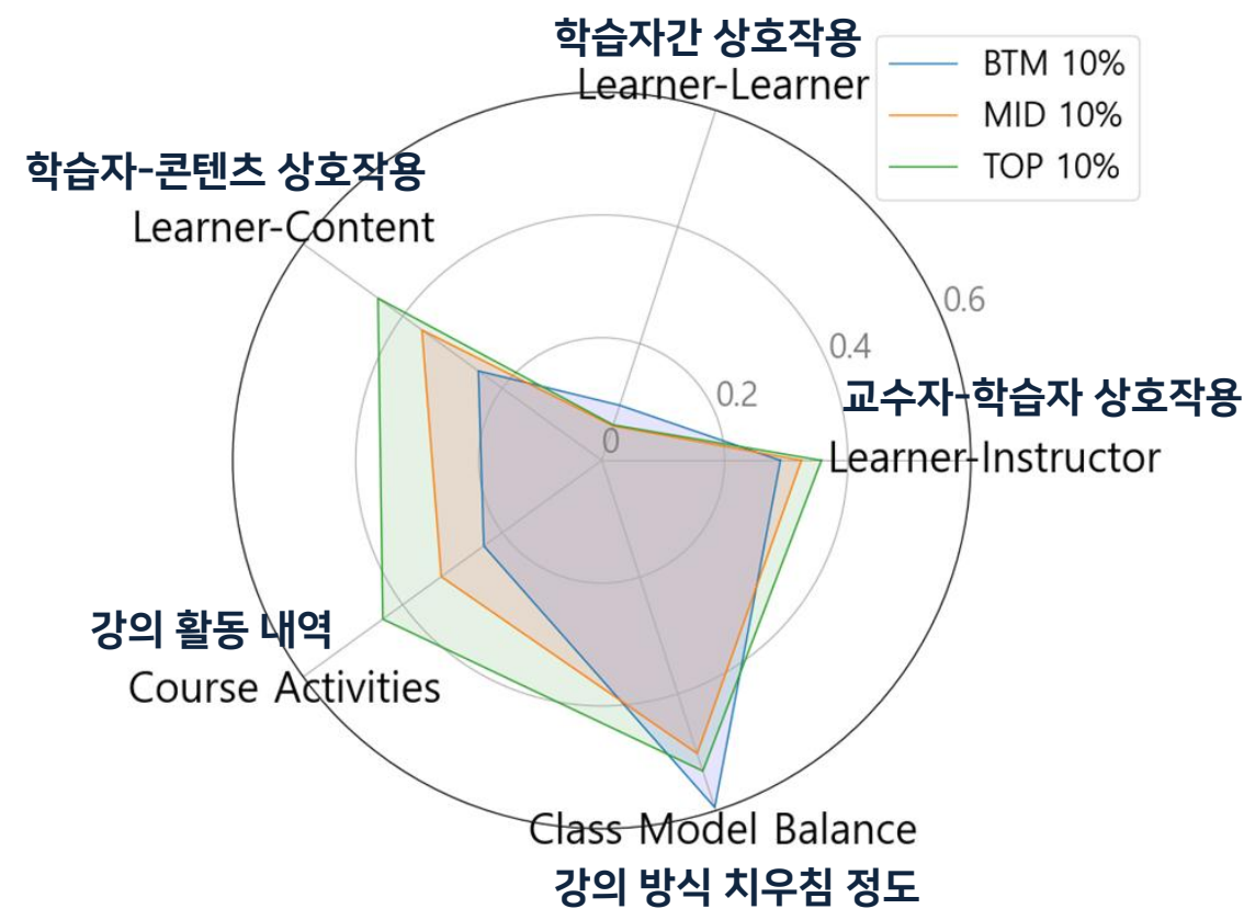
< 그림 3. 성적 등급별 학습자 상호 작용의 평균 >
