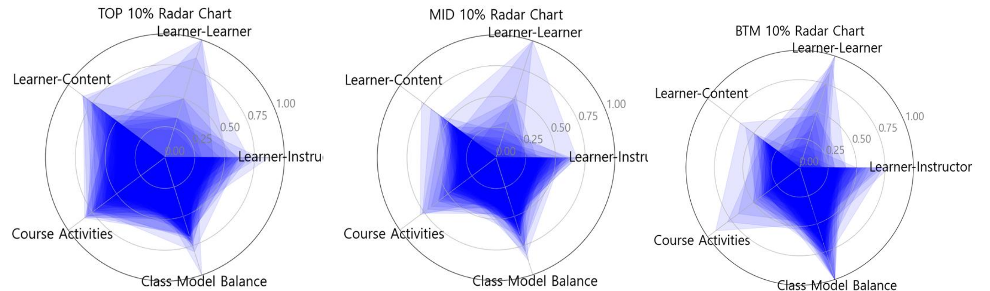
< 그림 4. 성적 등급별 학습자 상호 작용 방식형 중첩 차트 >
