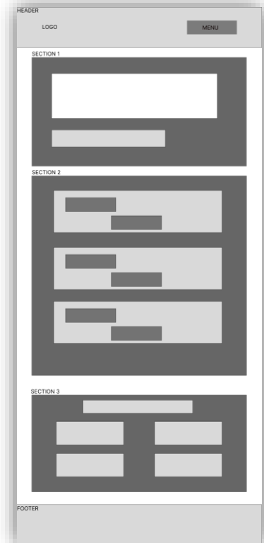
Hình 5. Layout Trang Vocabulary (Từ vựng) - Giao diện điện thoại (Mobile)
