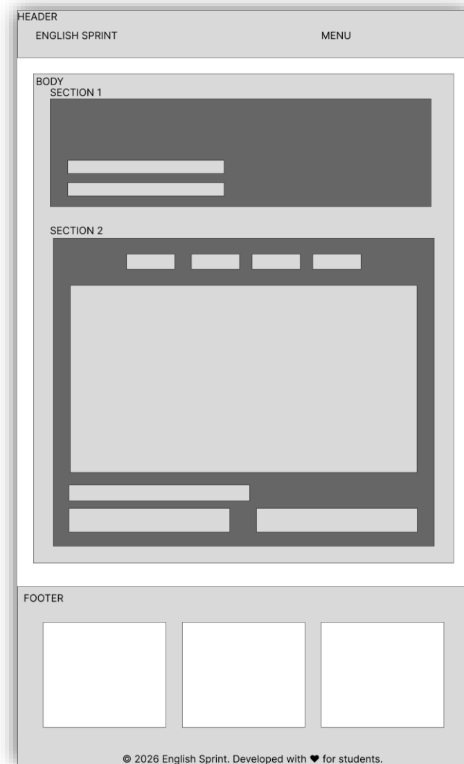
Hình 6. Layout Trang Grammar (Ngữ pháp) - Giao diện máy tính (Desktop)
