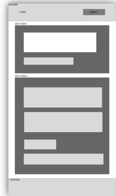
Hình 13. Layout Trang Progress (Tiến độ) - Giao diện điện thoại (Mobile)
