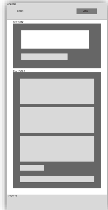
Hình 9. Layout Trang Reading (Đọc hiểu) - Giao diện điện thoại (Mobile)
