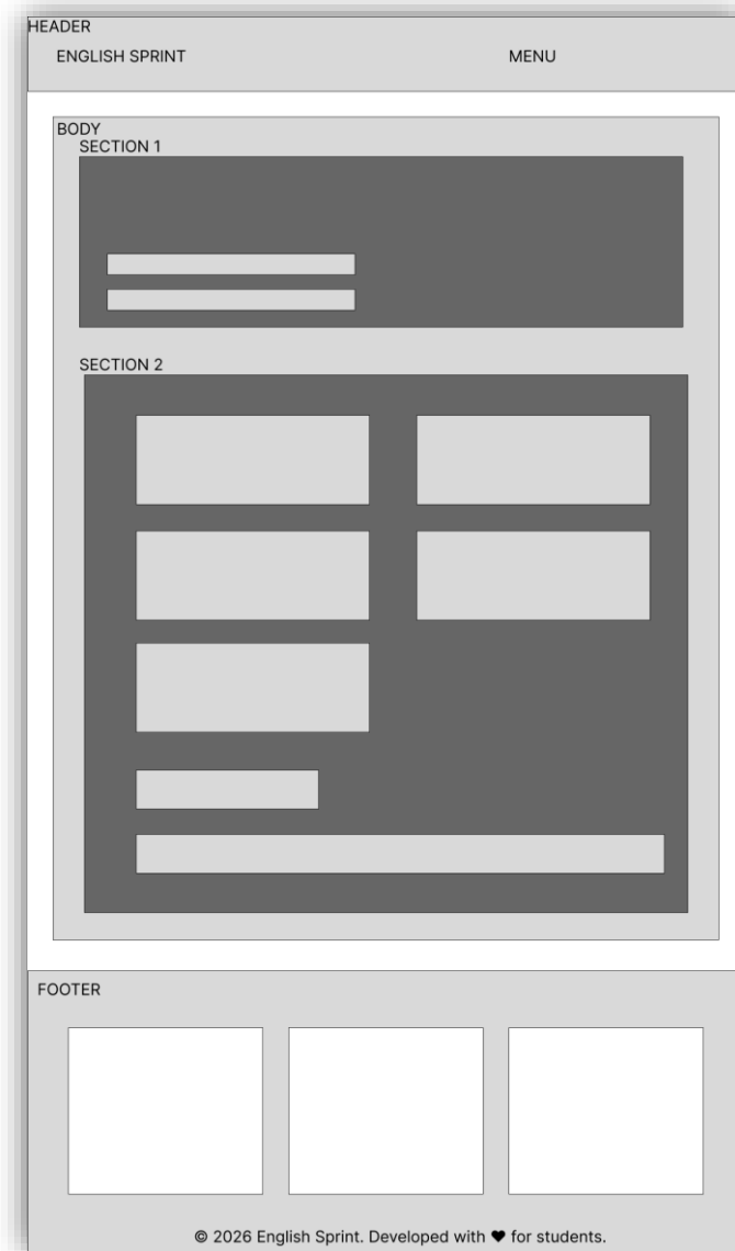
Hình 10. Layout Trang Quiz (Trắc nghiệm) - Giao diện máy tính (Desktop)
