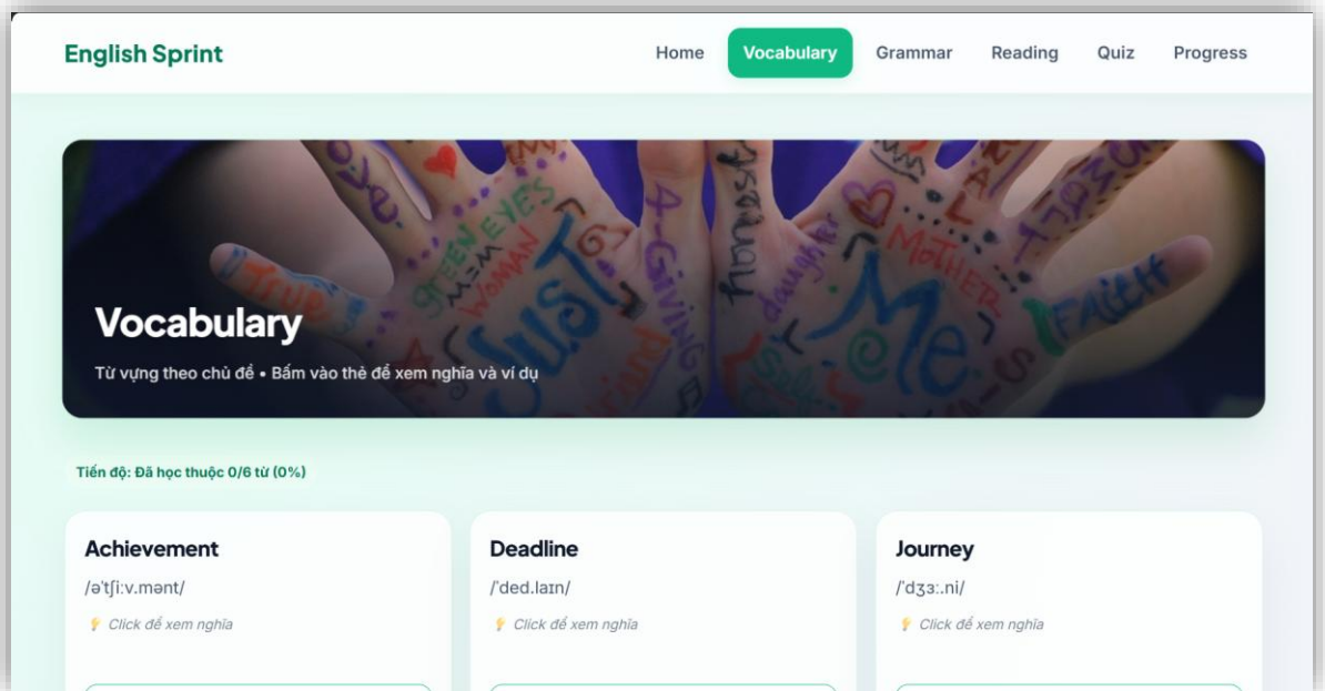
Hình 2. Giao diện Trang Vocabulary (Từ vựng)
